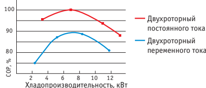
Энергоэффективность компрессора
