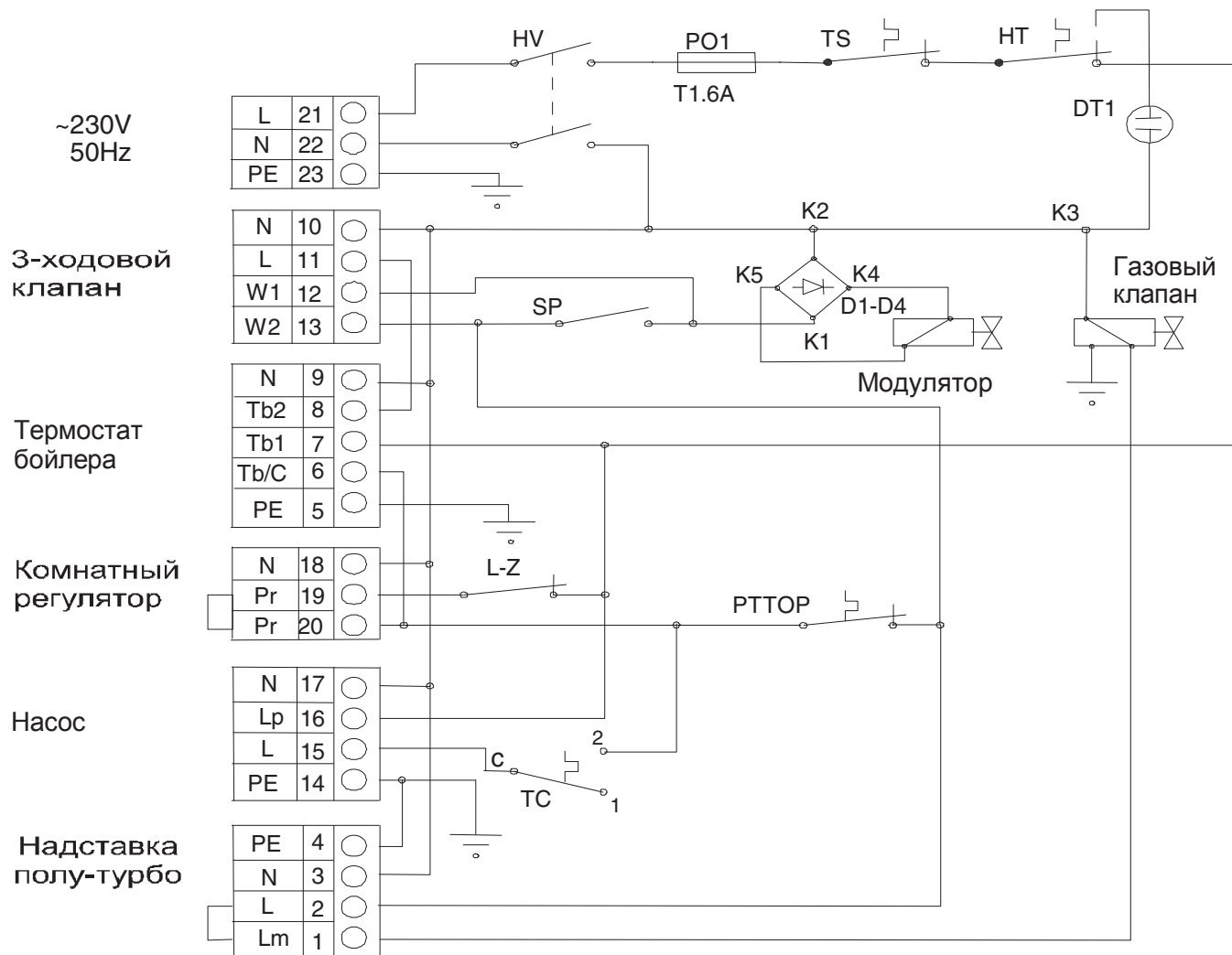
Рис. 5а – Схема электрического подключения котла 20, 30, 40, 50 PLO
