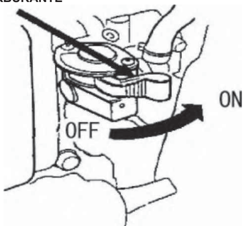
VALVOLA CARBURANTE
