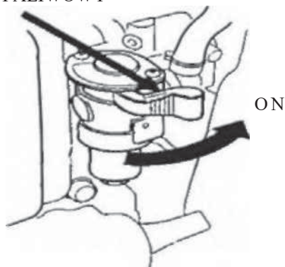
ZAWÓR PALIWOWY
