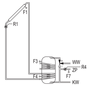
Дополнительная схема с Гидравлической схемой 1
