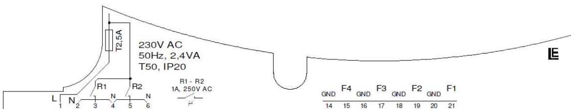
Схема подключений
