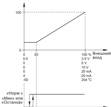
Рис. 47 «Линейная с мин. режимом»
