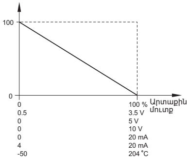
Նկար 48 «Հետադարձ գծային»
