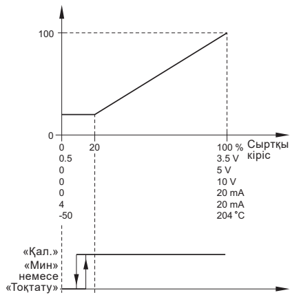
47-сурет «Мин режиммен сызықтық»
