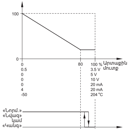
Նկար 49 «Հետադարձ՝ կանգով» և «Հետադարձ՝ նվազ. ռեժիմով»
