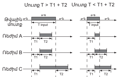
Նկար 42 Տևողության թայմերի գործառույթ թվային մուտքերի համար
