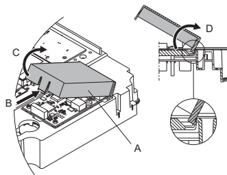
Рис. 64 Снятие крышки модуля СИМ
