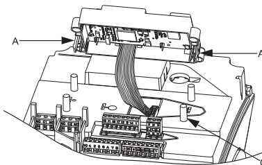
Рис. 60 Размещение пластмассовой крышки
