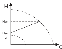
Пропорционалдуу басым
