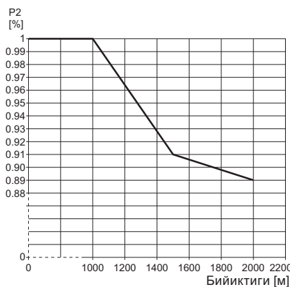
13-сүр. Электр кыймылдаткычынын чыгуу кубаттуулугунун деңиз деңгээлинен бийиктигине жараша төмөндөөсү (P2)
