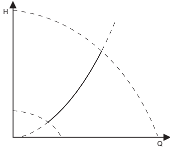
Նկար 35 «Մշտական մակարդակ»
