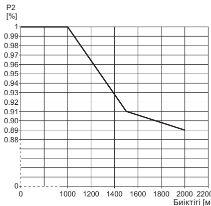
13-сурет Теңіз деңгейінен жоғары биіктігіне байланысты электр қозғалтқыштың (P2) шығыс қуатын төмендету
