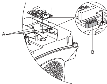
66-сурет SIM модулін орнату
