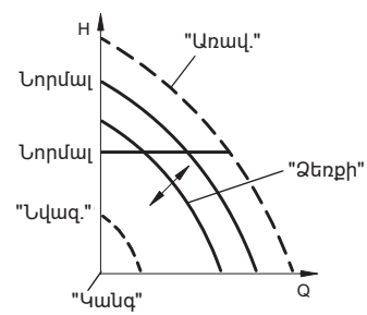
Նկար 22 Աշխատանքի ռեժիմներ
