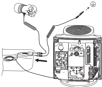
62-сурет Антистатикалық қызметтік жинақ
