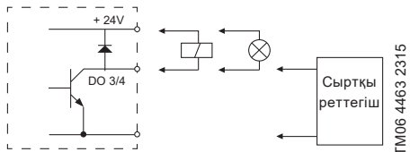
41-сурет Теңшелмелі сандық кірістер немесе шығыстар мысалы
