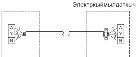
Сүрөт 11 3 жылкалуу экрандаштырылган кабелди туташтыруу
