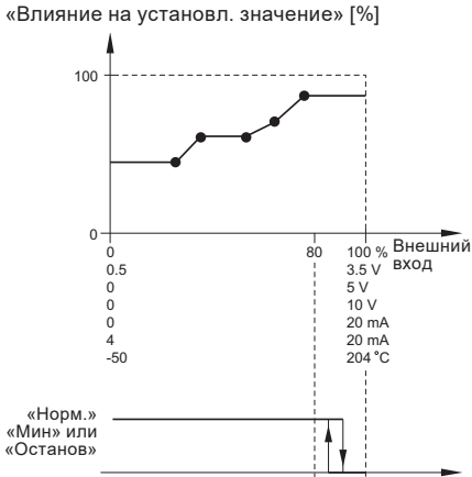
Рис. 52 «Таблица влиян. с остан. у макс.» (пример с пятью точками)
