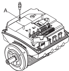
65-сурет Бекіту бұрандасын шешу
