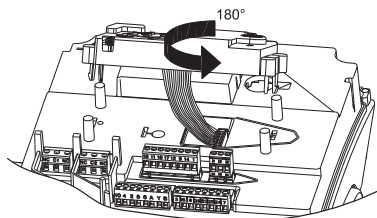
Рис. 59 Поворот пластмассовой крышки
