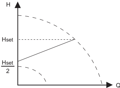
Рис. 23 «Пропорциональное давление»
