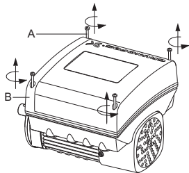
63-сурет Клеммалық қорап қақпағын шешу
