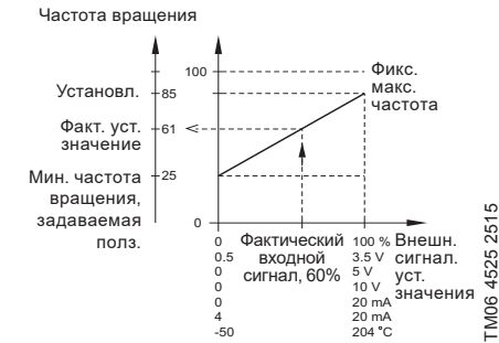
Рис. 45 Пример настройки регулирования установленного значения с постоянной характеристикой
