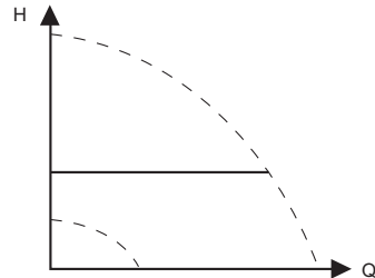
Рис. 25 «Постоянное давление»
