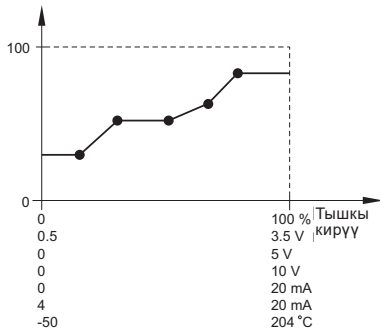
50-сүр. «Таасир этүү таасири» (беш чекит менен мисал)
