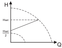
Пропорционалды қысым
