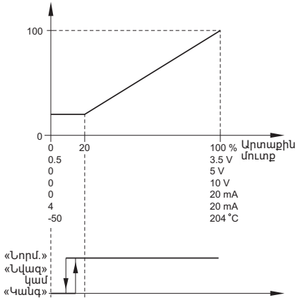
Նկար 47 «Գծային՝ նվազ. ռեժիմով»
