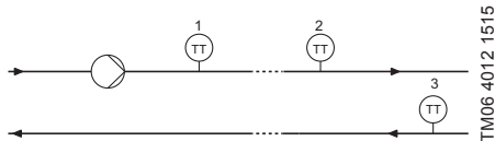
Նկար 39 PT100/1000 տվիչի տեղակայման ակնարկ
