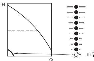
Рис. 18 Режим минимальной характеристики
