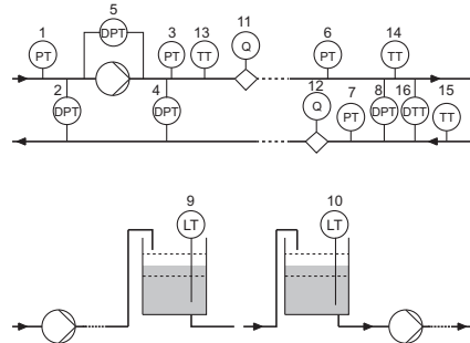
38-сүр. Көрсөткүчтүн жайгашкан ордунун сереби
