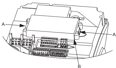
Рис. 58 Подъем пластмассовой крышки
