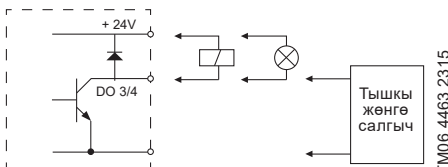
41-сүр. Тескелген санариптик кирүүлөрдүн же чыгуулардын мисалы
