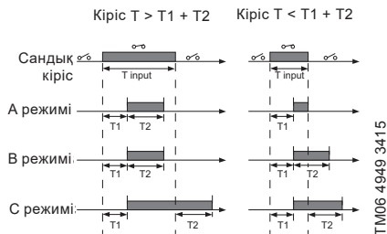
42-сурет Сандық кірістердің ұзақтық таймерінің функциясы
