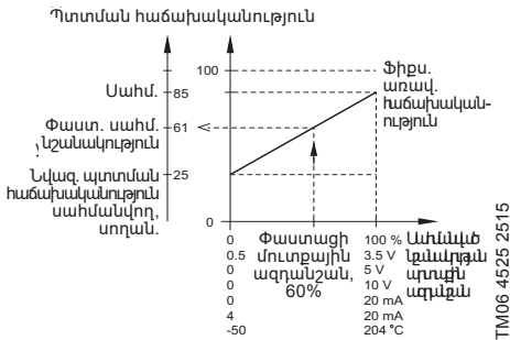
Նկար 45 Մշտական բնութագրով սահմանված նշանակության կարգավորման օրինակ
