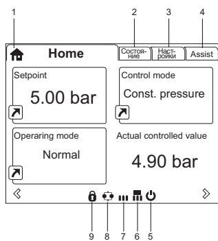
Рис. 20 Пример дисплея «Home»
