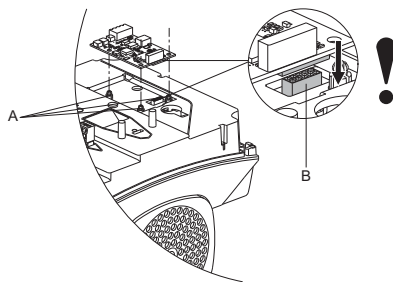
Рис. 66 Установка модуля СИМ
