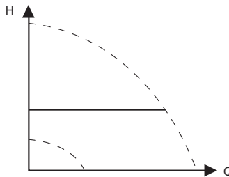
Рис. 29 «Постоянный перепад давления»
