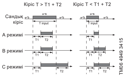
40-сурет Сандық кірістердің ұзақтық таймерінің функциясы
