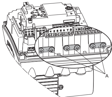
67-сурет Кабельдердің экрандалған орамдарын жерге түйықтау
