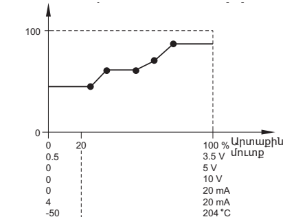
«Ազդեցություն սահմանված նշանակության վրա» [%]
