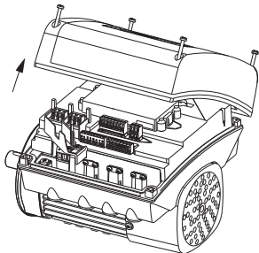
Рис. 57 Снятие крышки клеммной коробки
