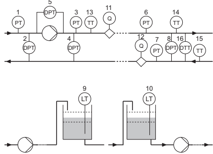
Նկար 38 Տվիչի տեղակայման ակնարկ
