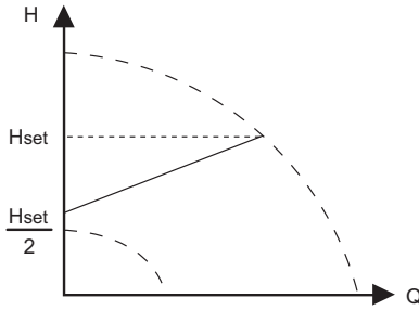
23-сурет «Пропорционалды қысым»
