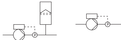
Рис. 26 «Постоянное давление»
