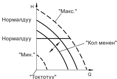
22-сүрөт Иштөө режим
