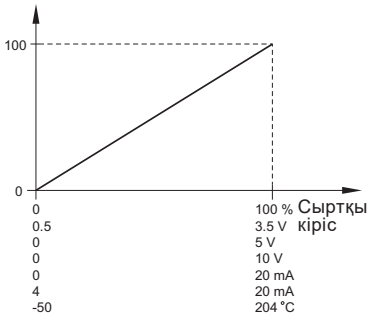
46-сурет «Сызықтық»
