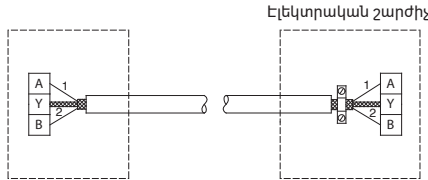
Նկար 12 2-ջիղանի վահանավորված մալուխի միացում
