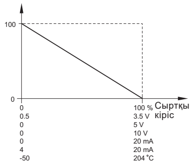
48-сурет «Кері сызықтық»
