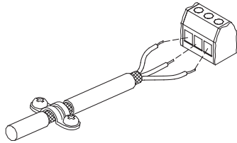
10-сүр. Экраны жана өткөргүч туташуулары менен тазаланган кабел
