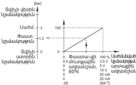
Նկար 44 Սահմանված նշանակության ըստ տվիչների ազդանշանների փոփոխության օրինակ
