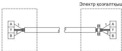
12-сурет 2 тарамды қоршалған кабельді қосу
