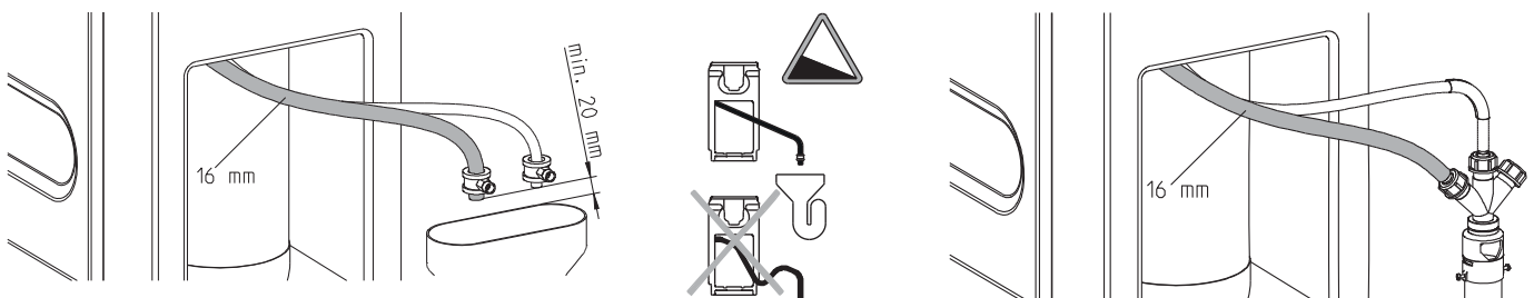
Abb. D-4: Kanalanschluss Überlaufschlauch Salztank mit und ohne Kanalanschluss DN 50 nach DIN EN 1717 für Kleinenthärtungsanlagen (Bestell-Nr. 187 840)
