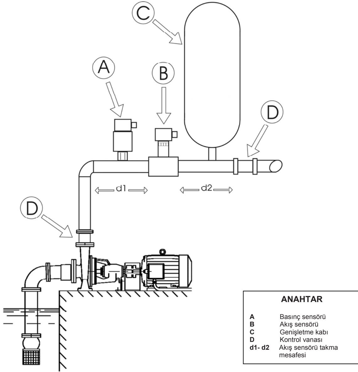
Şekil 4: Hidrolik kurulum
