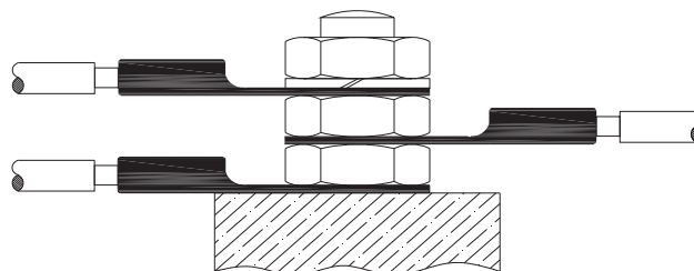
Figura 3: Conexión del conductor de tierra
