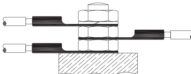
Σχήμα 3: Σύνδεση του αγωγού γείωσης
