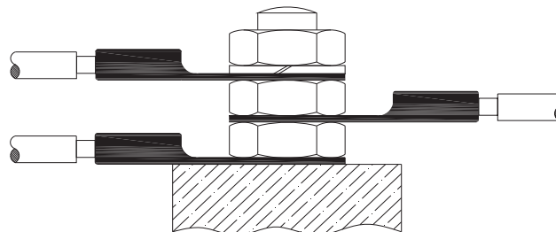
Fig. 3: Anslutning av jordledare
