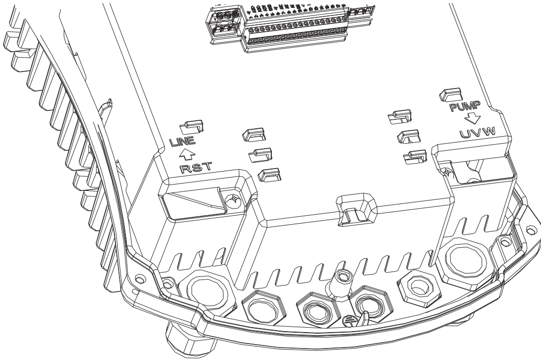
Şekil 2: Elektrik bağlantıları
