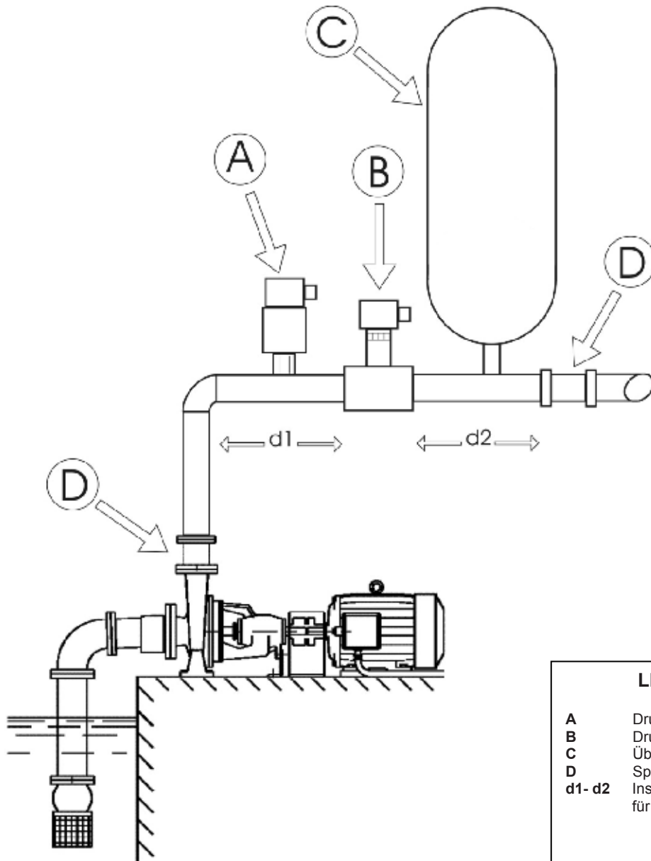
Abbildung 4: Hydraulik-Installation
