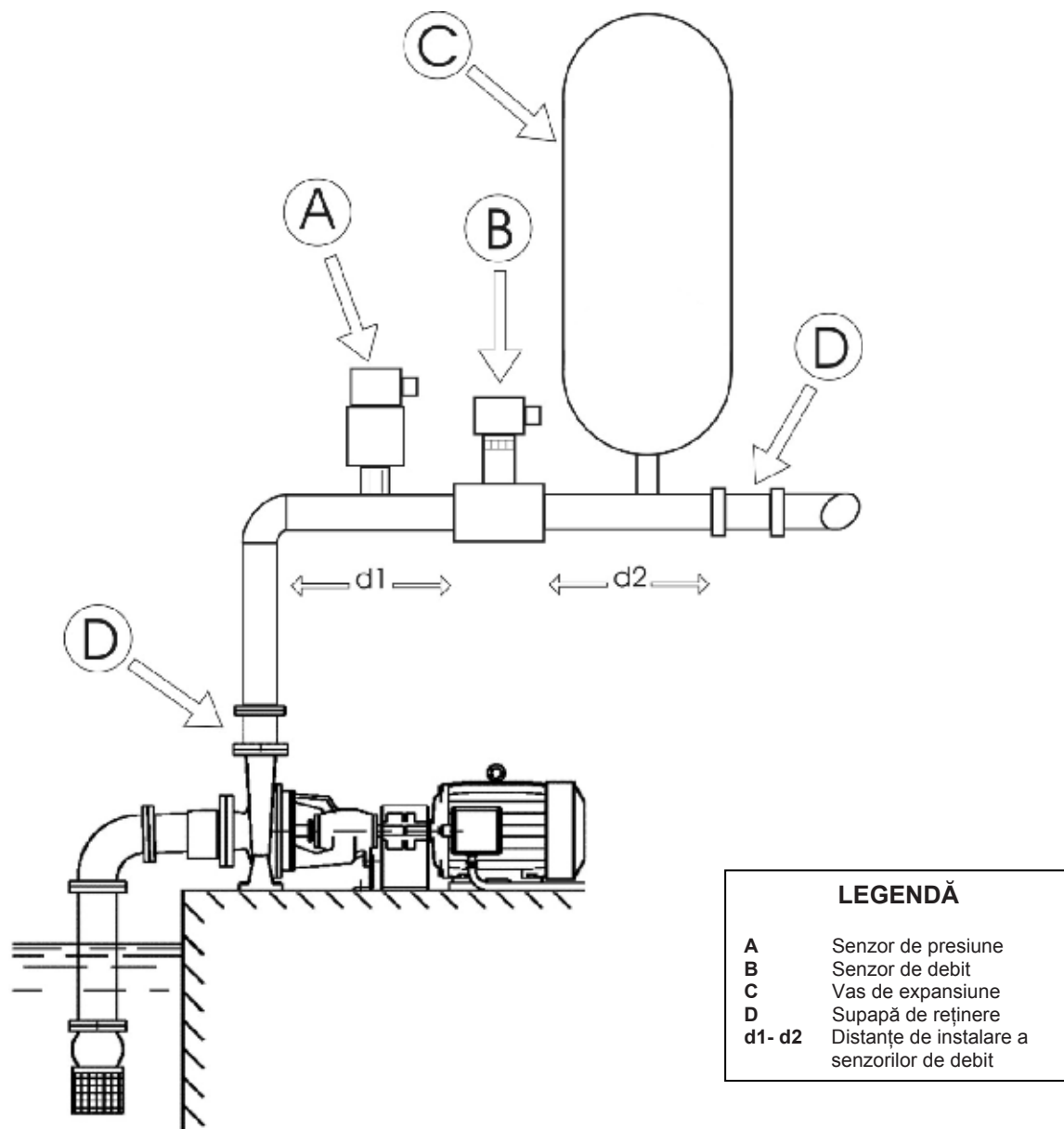
Figura 4: Instalația hidraulică
