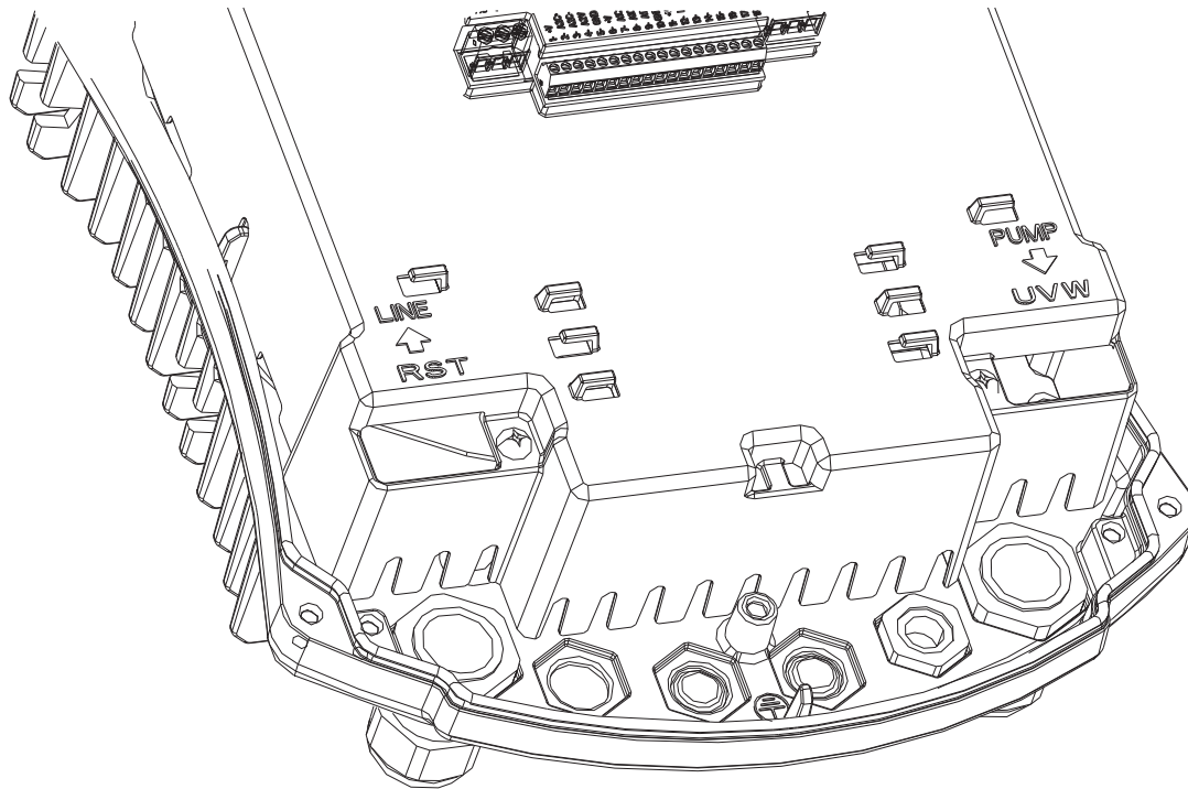
Figura 2: Conectări electrice
