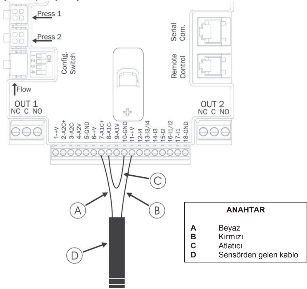
Şekil 6: - 20 mA basınç sensörünü bağlama
