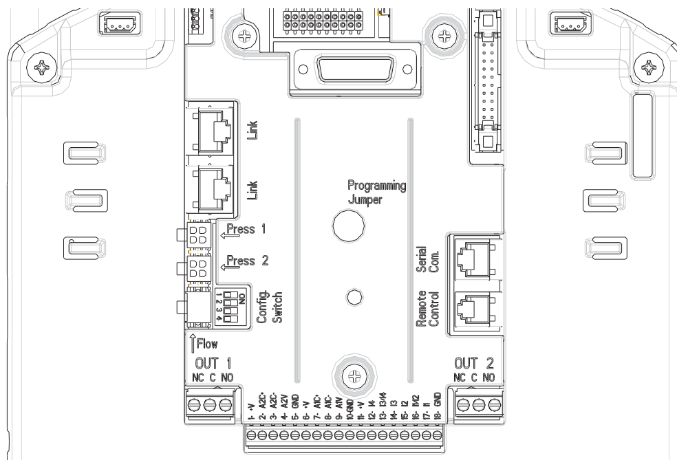
Afbeelding 5: aansluitingen
