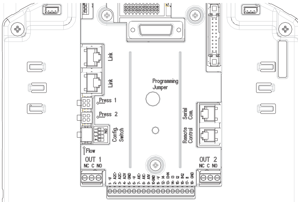
Abbildung 5: Anschlüsse
