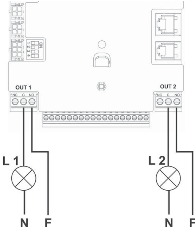
Şekil 7: bağlantıları örneği
