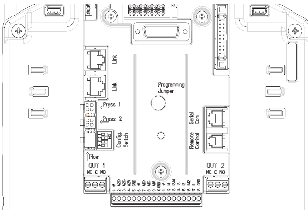
Figura 5: Connessioni
