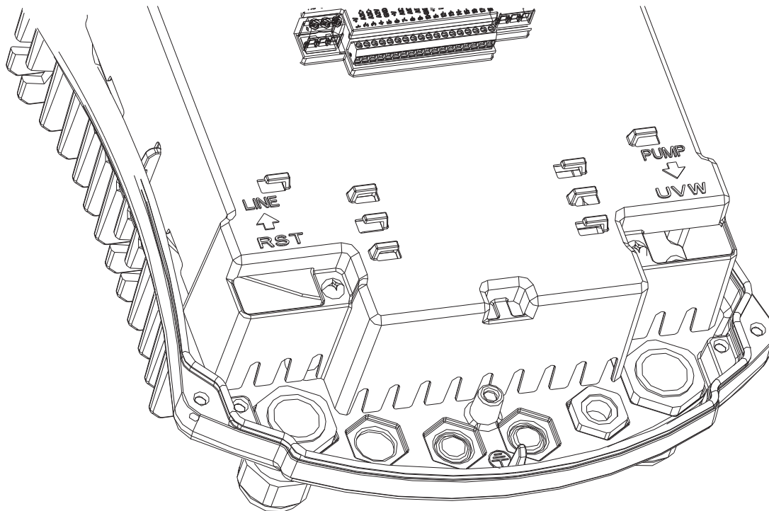
Abbildung 2: Elektrische Anschlüsse
