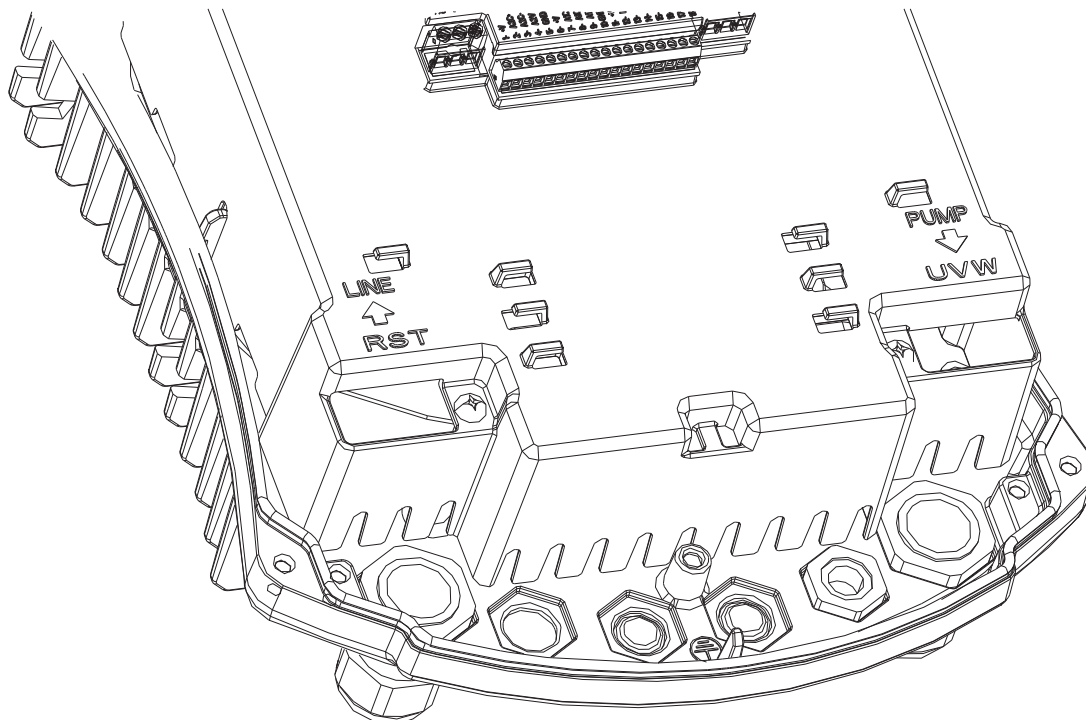
Figure 2: Connexions électriques
