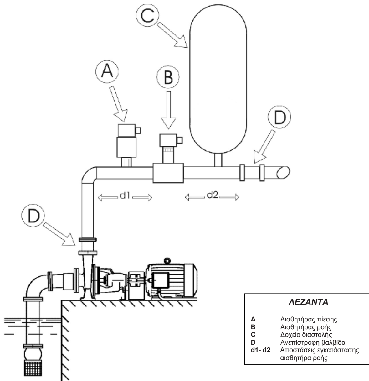
Σχήμα 4: Υδραυλική εγκατάσταση
