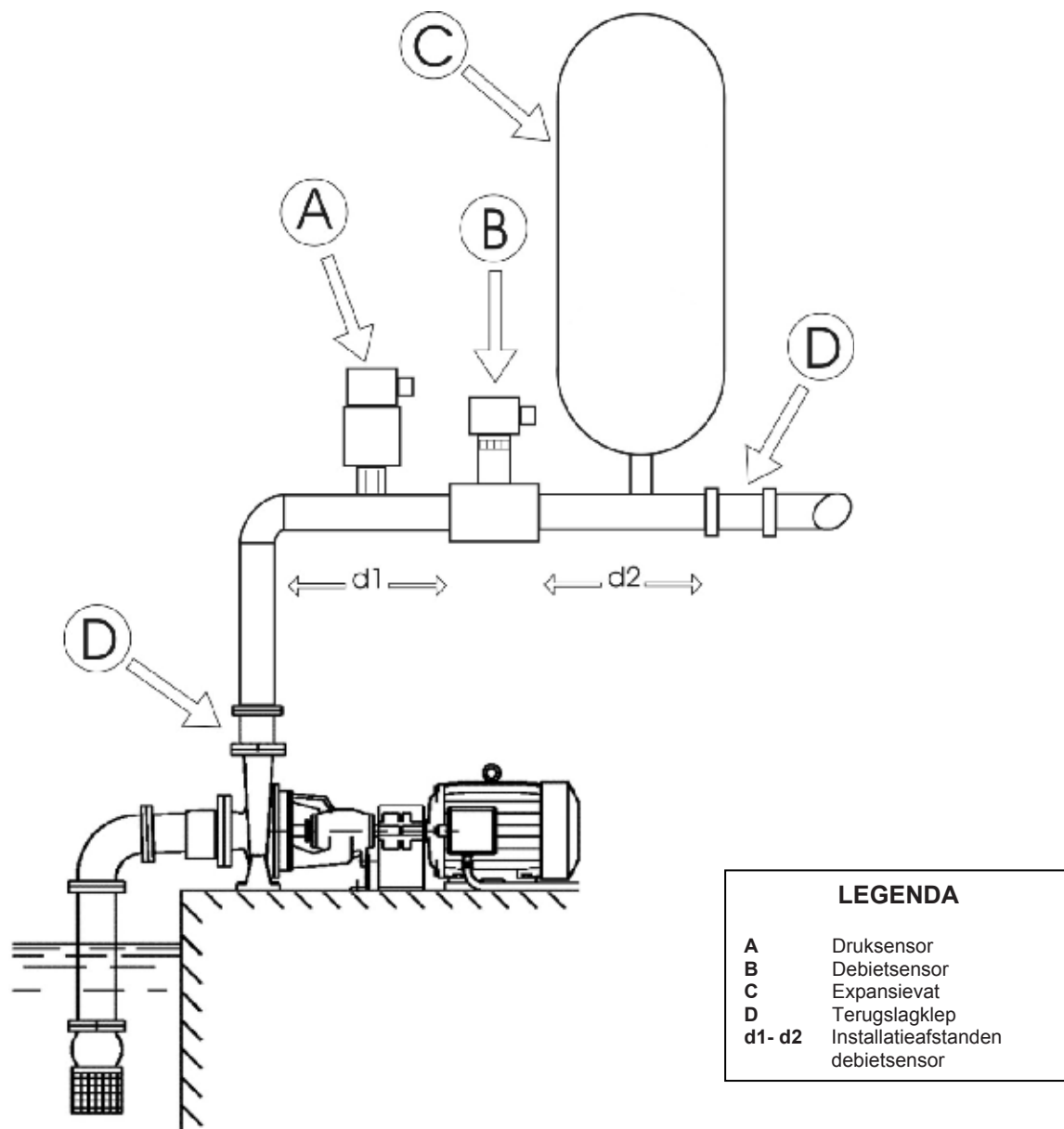
Afbeelding 4: hydraulische installatie
