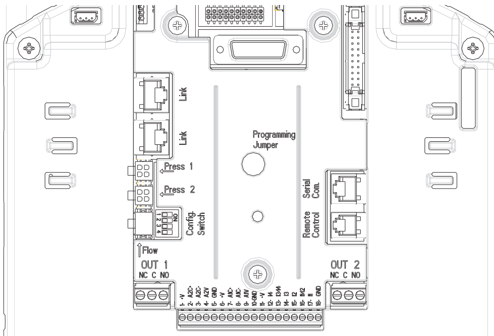
Рисунок 5: Соединения
