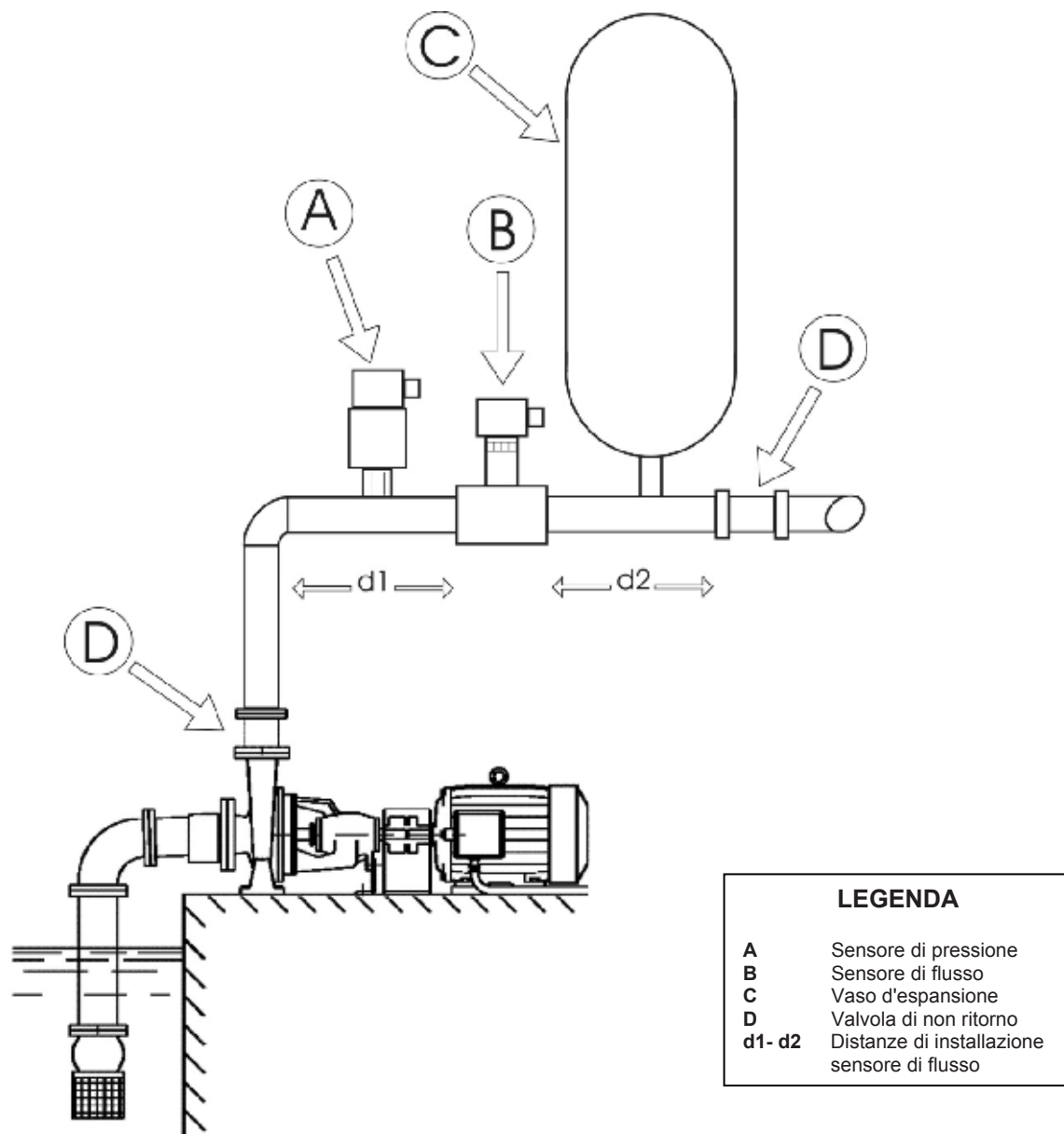
Figura 4: Installazione idraulica
