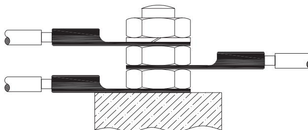
Afbeelding 3: Aansluiting van de aardgeleider
