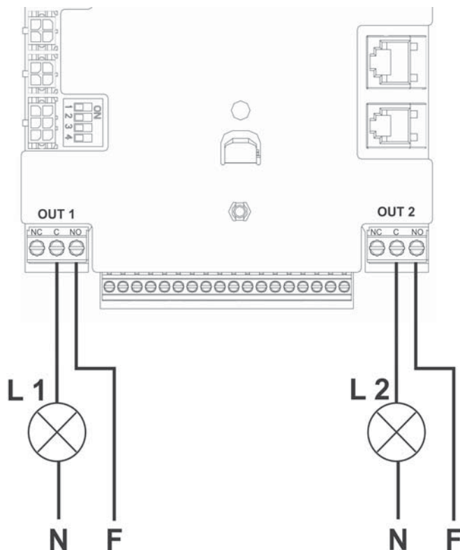
Abbildung 7: Anschlussbeispiel der Ausgänge
