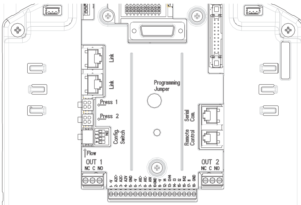
Figura 5: Conexiones
