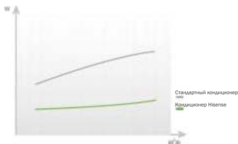
Расход воздуха – Энергопотребление
