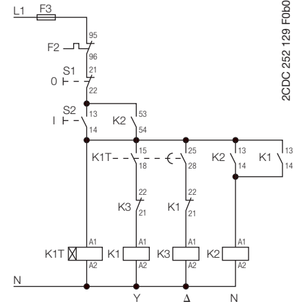
Схема управления
