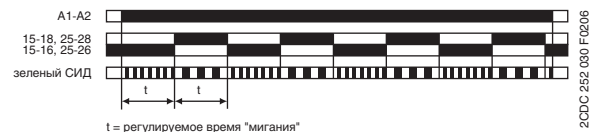
t = регулируемое время “мигания”
