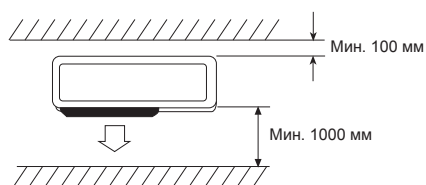
Размещение наружного блока с препятствиями спереди и сзади
