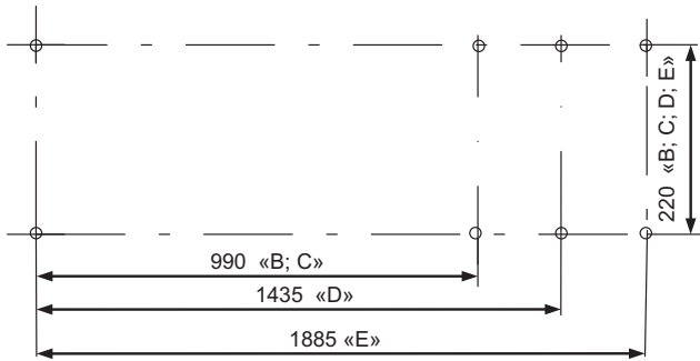
Рис. 6. Схема сверления отверстий под анкерные болты для дозировочных установок DSS
