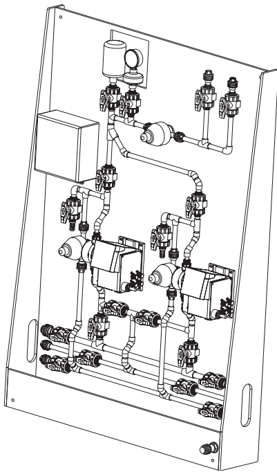
Рис. 2. Дозировочная установка DSS с одним рабочим и одним резервным насосами* (компоновка C)
