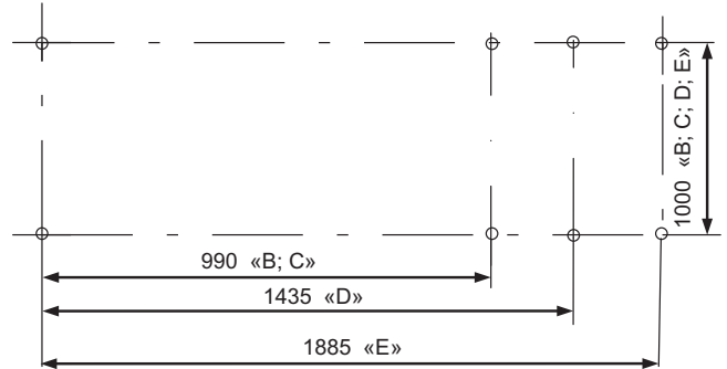
Рис. 8. Схема сверления отверстий для крепления дозировочных установок DSS на стене
