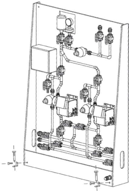
Рис. 7. Монтаж дозировочной установки DSS на полу
