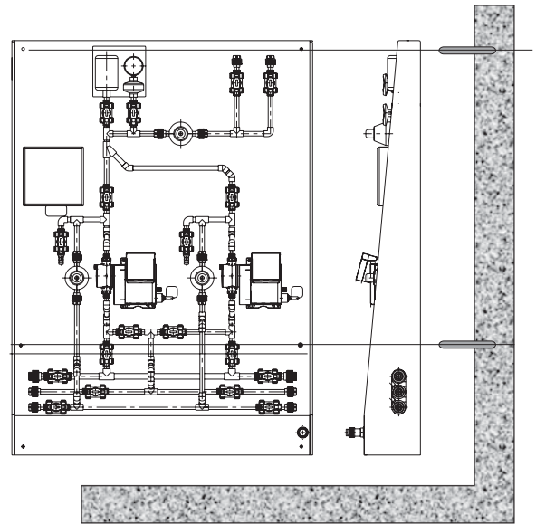
Рис. 9. Монтаж дозировочной установки DSS на стене
