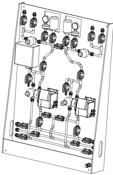
Рис. 1. Дозировочная установка DSS с двумя рабочими насосами* (компоновка B)
