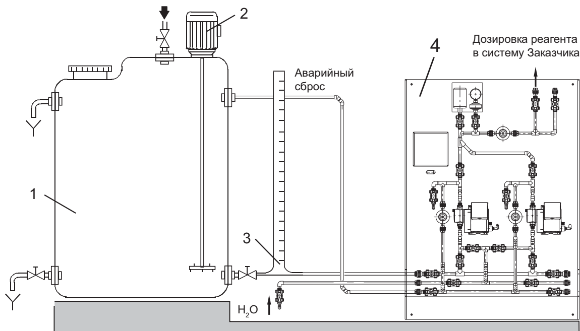
Рис. 10. Типовая схема монтажа и подсоединения дозировочной установки DSS 1 - Дозировочная ёмкость, 2 – Перемешивающее устройство, 3 - Калибровочный цилиндр, 4 - Дозировочная установка DSS
