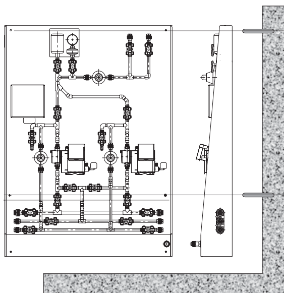
9-сур. DSS мөлшерлеу қондырғысын қабырғада орнату
