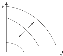
Рис. 38 "Постоянная характеристика"
