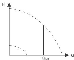
Рис. 34 Постоянный расход
