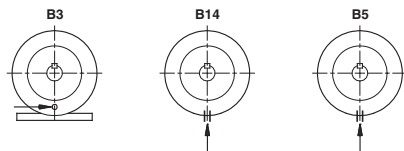
Рис. 3 Сливные отверстия
