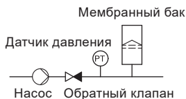
Рис. 54 Положение обратного клапана и датчика давления в системе с положительным давлением на входе
