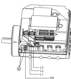
Рис. 7 Подключение к сети трёхфазных электродвигателей
