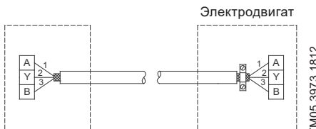
Рис. 11 Подключение 3-жильного экранированного кабеля
