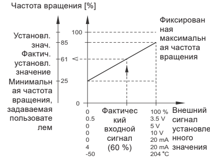
Рис. 46 Пример влияния установленного значения на постоянную характеристику
