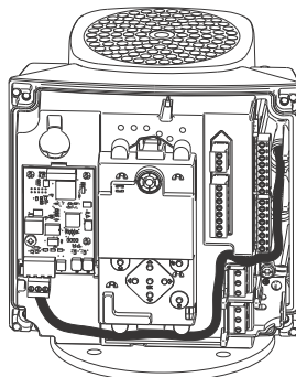
Рис. 64 Пример проводки
