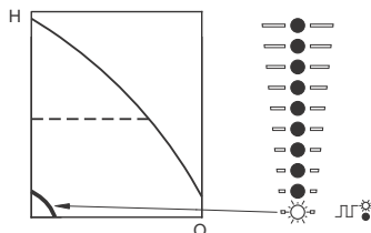
Рис. 20 Эксплуатация при минимальной характеристике
