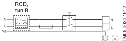
Рис. 4 Пример подключения к сети электродвигателя с выключателем электропитания, резервным плавким предохранителем и дополнительной защитой
