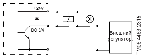
Рис. 42 Пример настраиваемых цифровых входов/выходов
