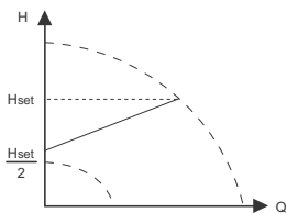
Рис. 25 "Пропорциональное давление"
