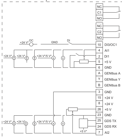
Рис. 9 Клеммы соединений, насосы CME (по заказу для насосов CRE, CRIE, CRNE, SPKE и MTRE)
