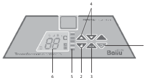
Рис. 2 Панель управления
