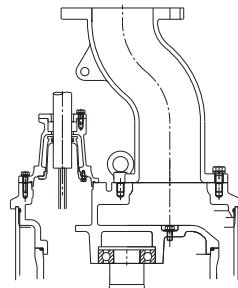
Фланцевое соединение
