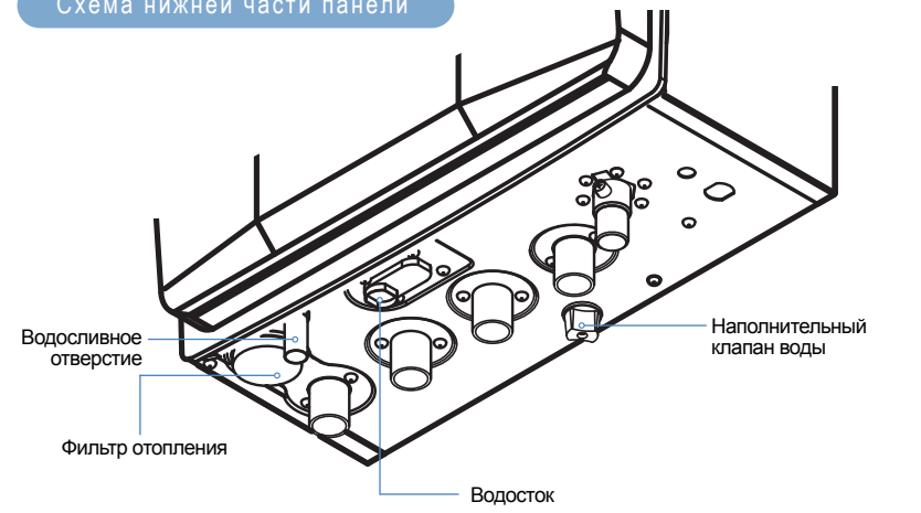
Схема нижней части панели
