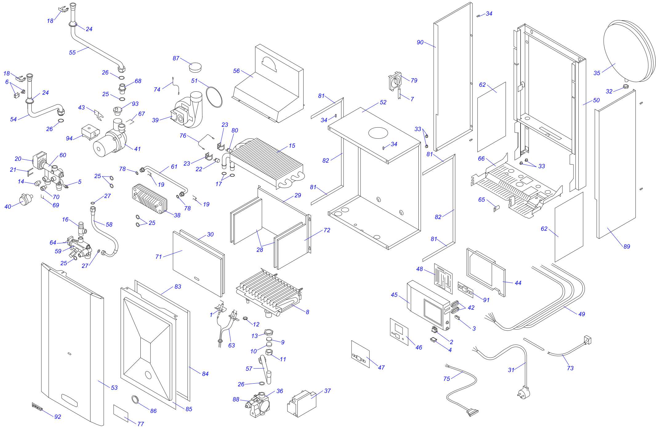
Навесные котлы
