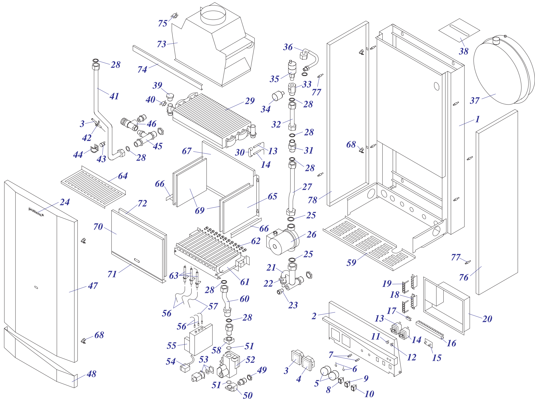
Навесные котлы
