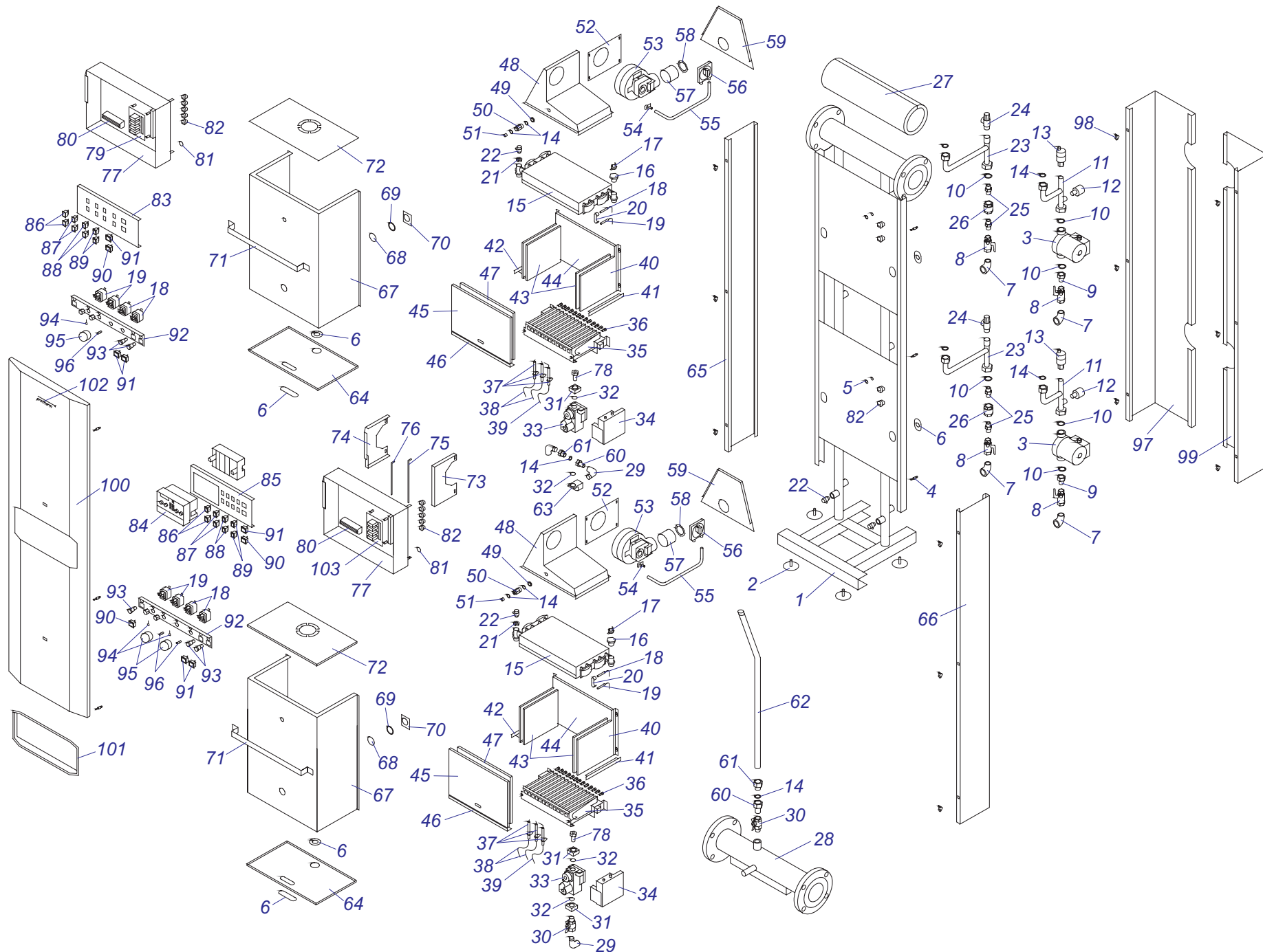
Напольные котлы
