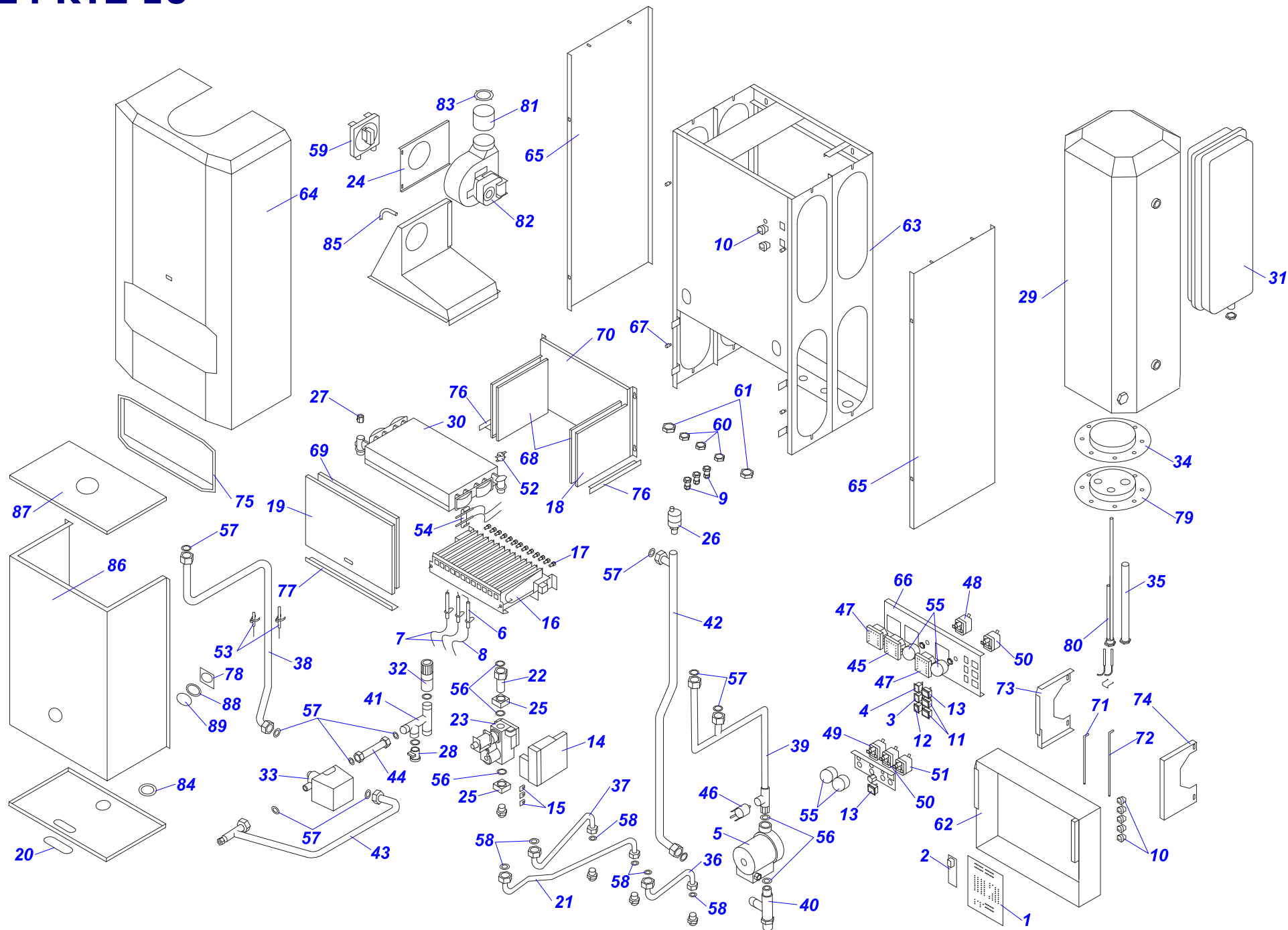
Навесные котлы
