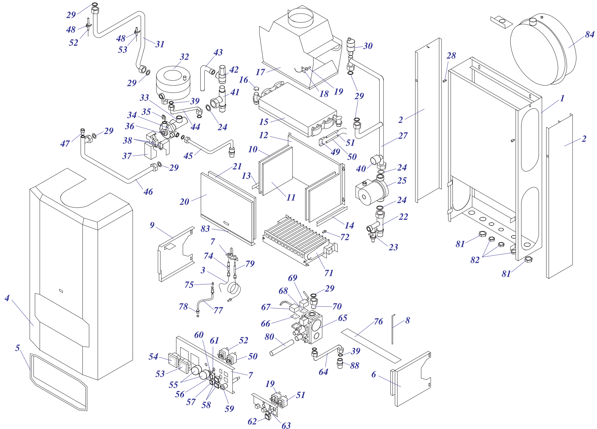
Навесные котлы
