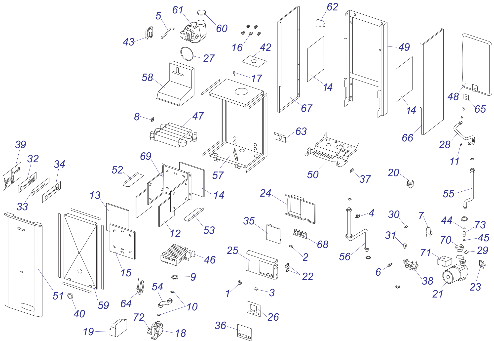
Навесные котлы
