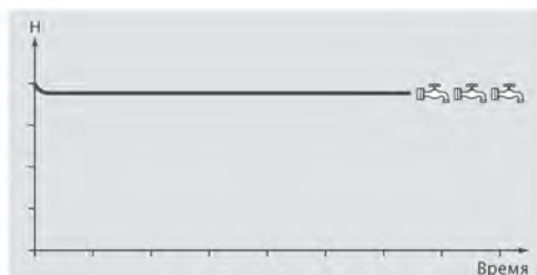
Работа TECNOPLUS – стабильное давление в системе при изменяющемся расходе воды.
