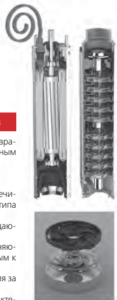
Ступень «плавающей» гидравлики
