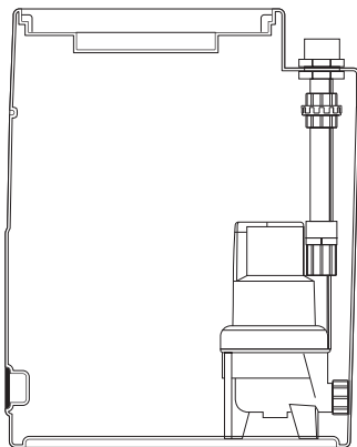
Комплект обвязки для установки DRAINBOX 300 1200 M D TP FL
