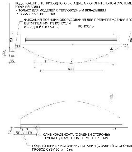
ВИД СНИЗУ
