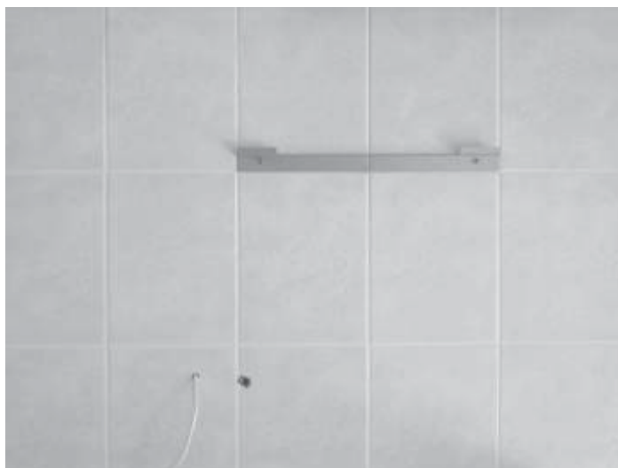
Пример подготовки к подключению прибора к электросети, слива конденсата и монтажа консоли.
