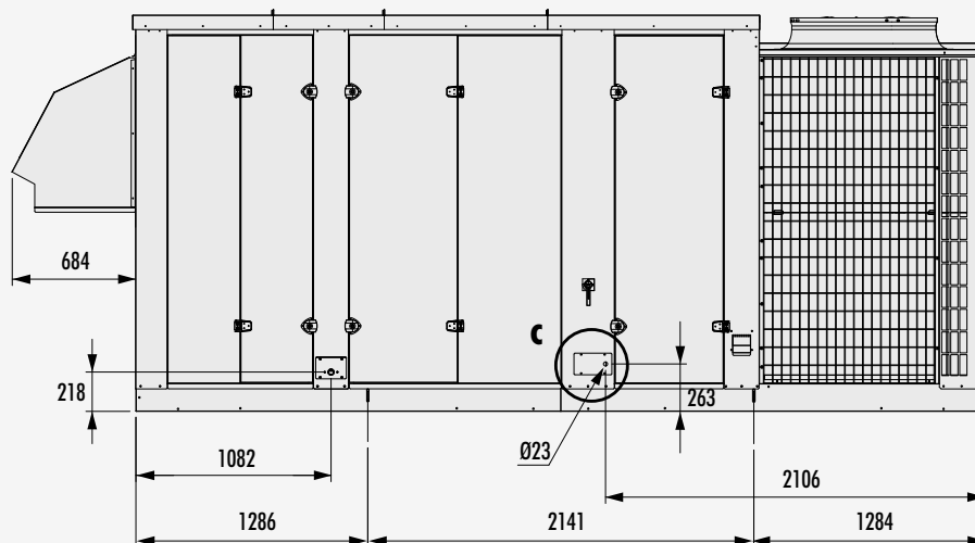
Детализовка C
