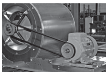
Индивидуальная платформа электродвигателя с регулирующим винтом
