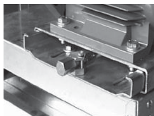
Индивидуальная платформа электродвигателя с регулирующим винтом
