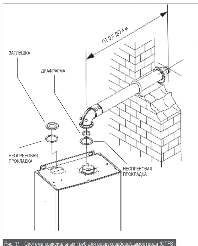
Рис. 11 - Система коаксиальных труб для воздухозабора/дымоотвода (СТФС)
