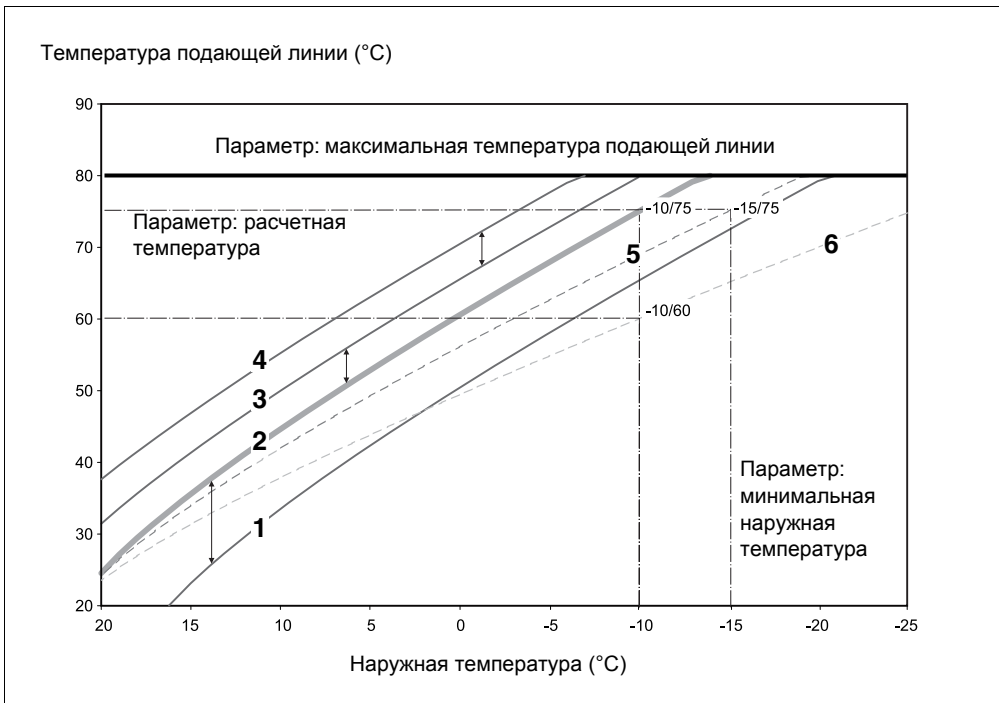
Рис. 11 Отопительная кривая для отопительной системы "Отопительный прибор"
