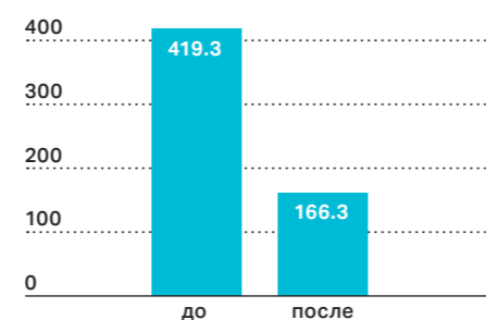
Потребление энергии в процессе производства в ватт-часах на метр трубы Merla
