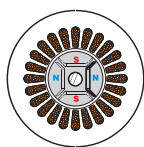
Централизованная обмотка
