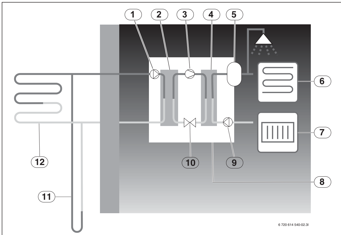
Рис 2 Принцип действия
