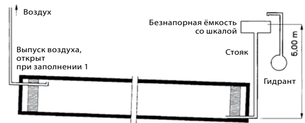
Рис. 10 Проверка герметичности
