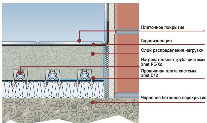
Гидроизоляция от поверхностных вод (влажные помещения)
