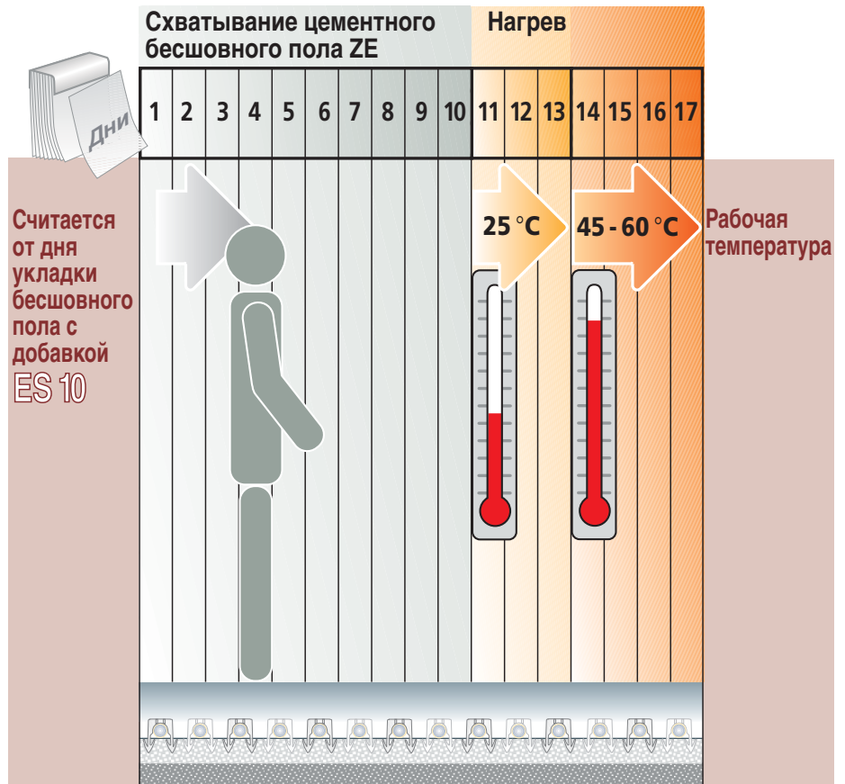
Время схватывания и прогрева для цементного бесшовного пола с добавкой ES 10
