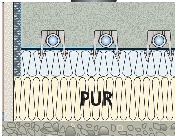
Прошивная плита системы xnet C12 NM 30-2
