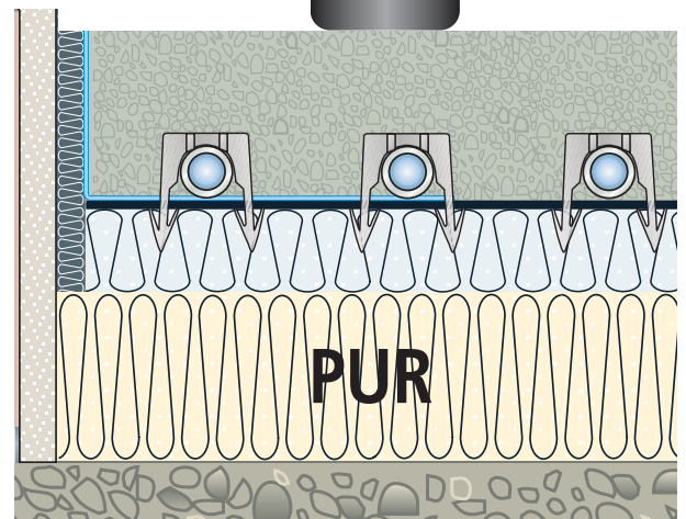
Прошивная плита системы xnet C12 NM 25-2
