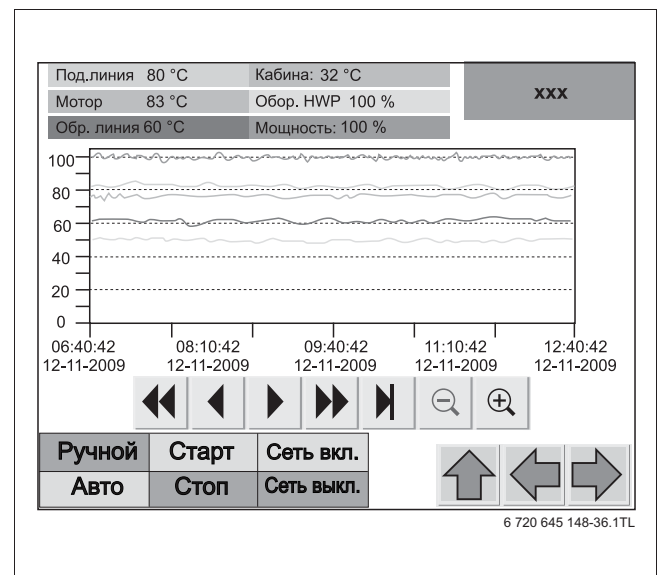
Рис. 49 Диаграмма «Температуры блок-ТЭС»
