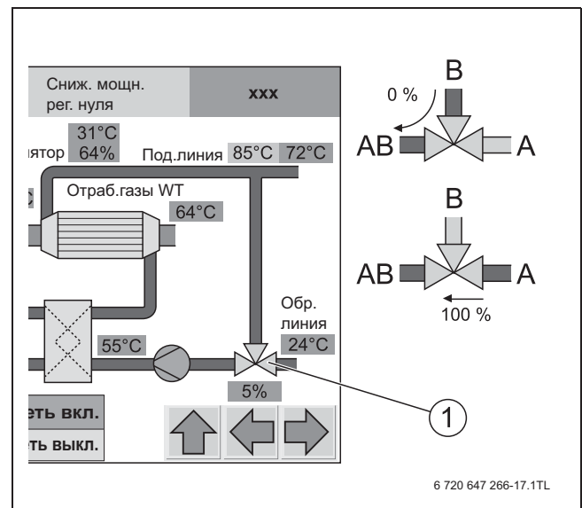
Рис. 53 Потоки через трёхходовой клапан
