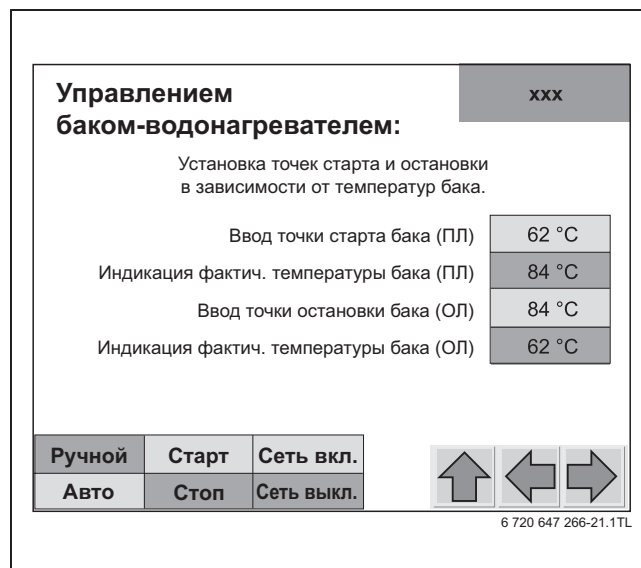
Рис. 40 Экран настройки «Управление бойлером»
