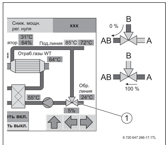
Рис. 36 Поток через трёхходовой клапан
