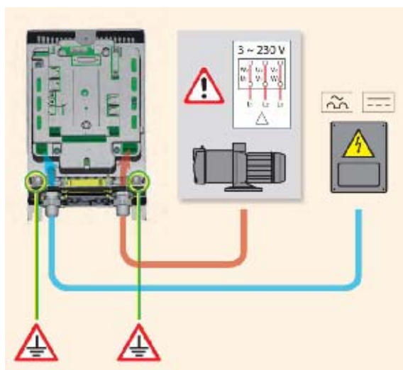
Fig. 5: Anslutning av pump AD 2.2 AC - 1.5 AC - 1.0 AC
