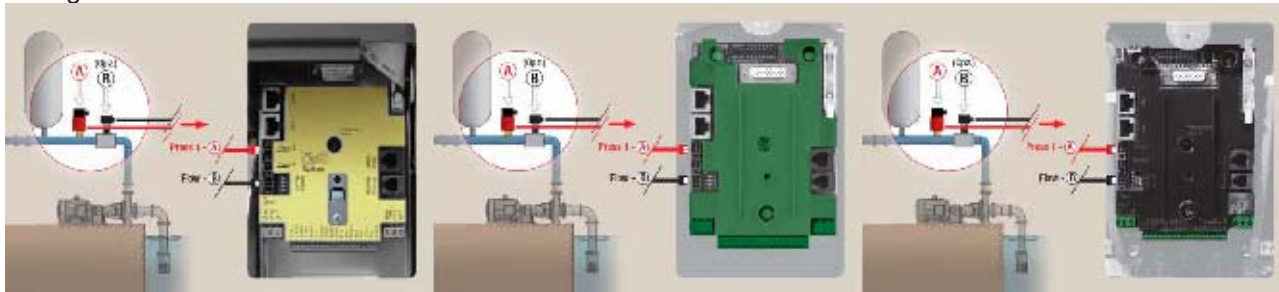
Fig. 7: Anslutning av sensorer
