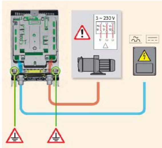
Şekil 5: AD 2.2 AC - 1.5 AC - 1.0 AC pompa bağlantısı
