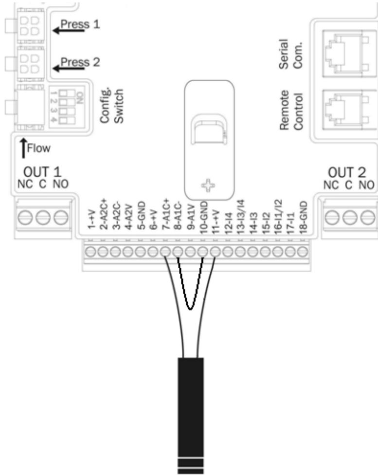
8.ábra: Nyomás szenzor bekötése 4 - 20mA
