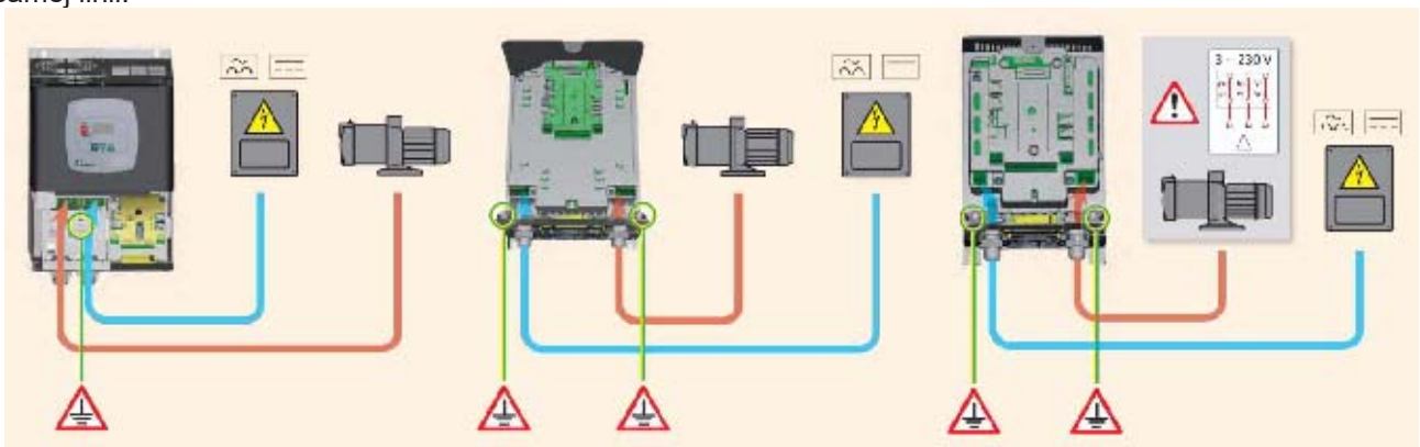
Rys. 4: Podłączenia elektryczne
