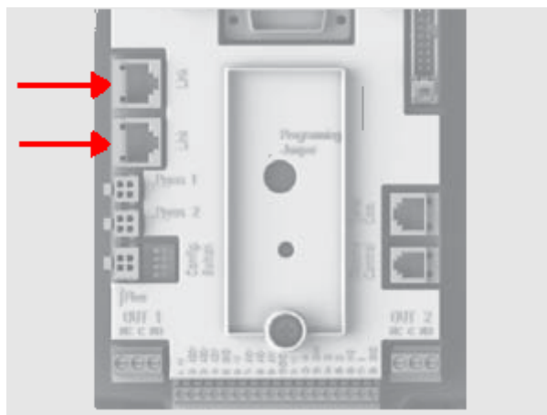
Figura 16: Conexión Link
