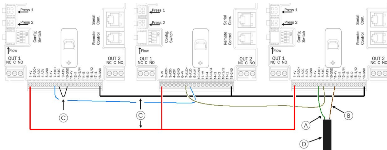
Figura 9: Conectarea senzorului de presiune 4 - 20 mA într-un sistem multi invertere
