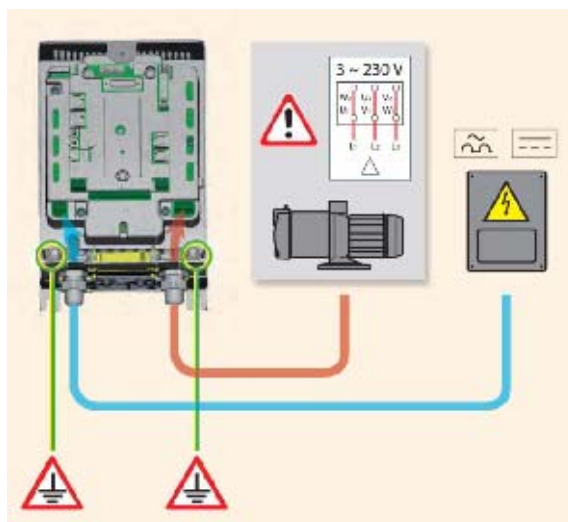
5.ábra: Szivattyú bekötés / AD 2.2 AC - 1.5 AC - 1.0 AC
