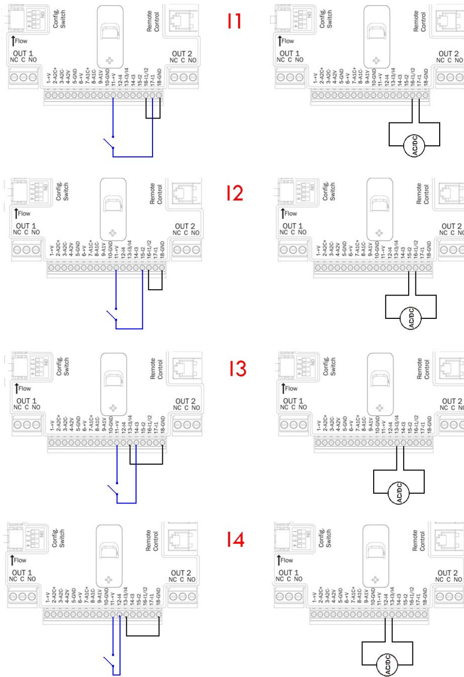
Рисунок 11: Пример соединения входов
