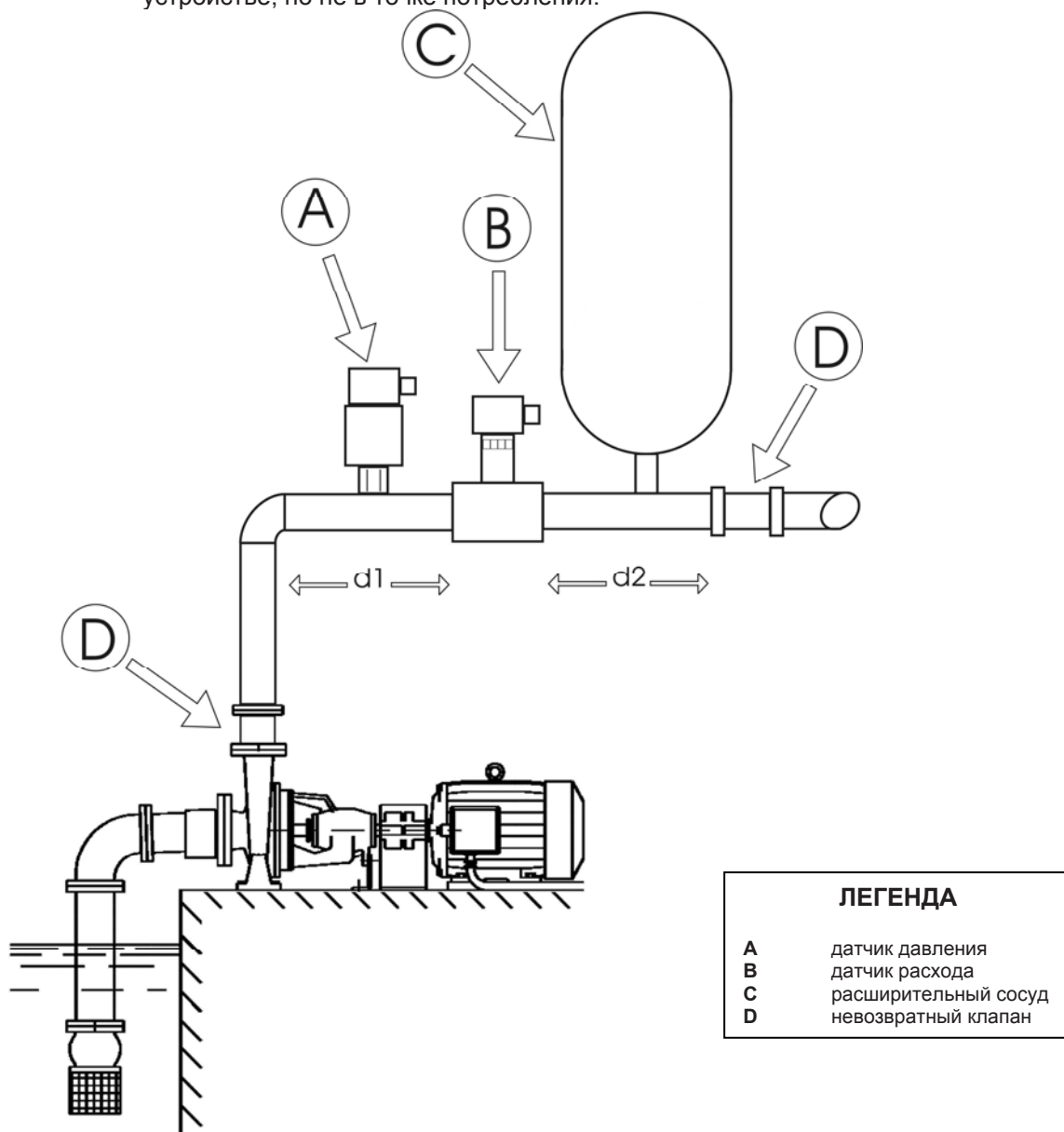
Рисунок 6: Гидравлический монтаж
