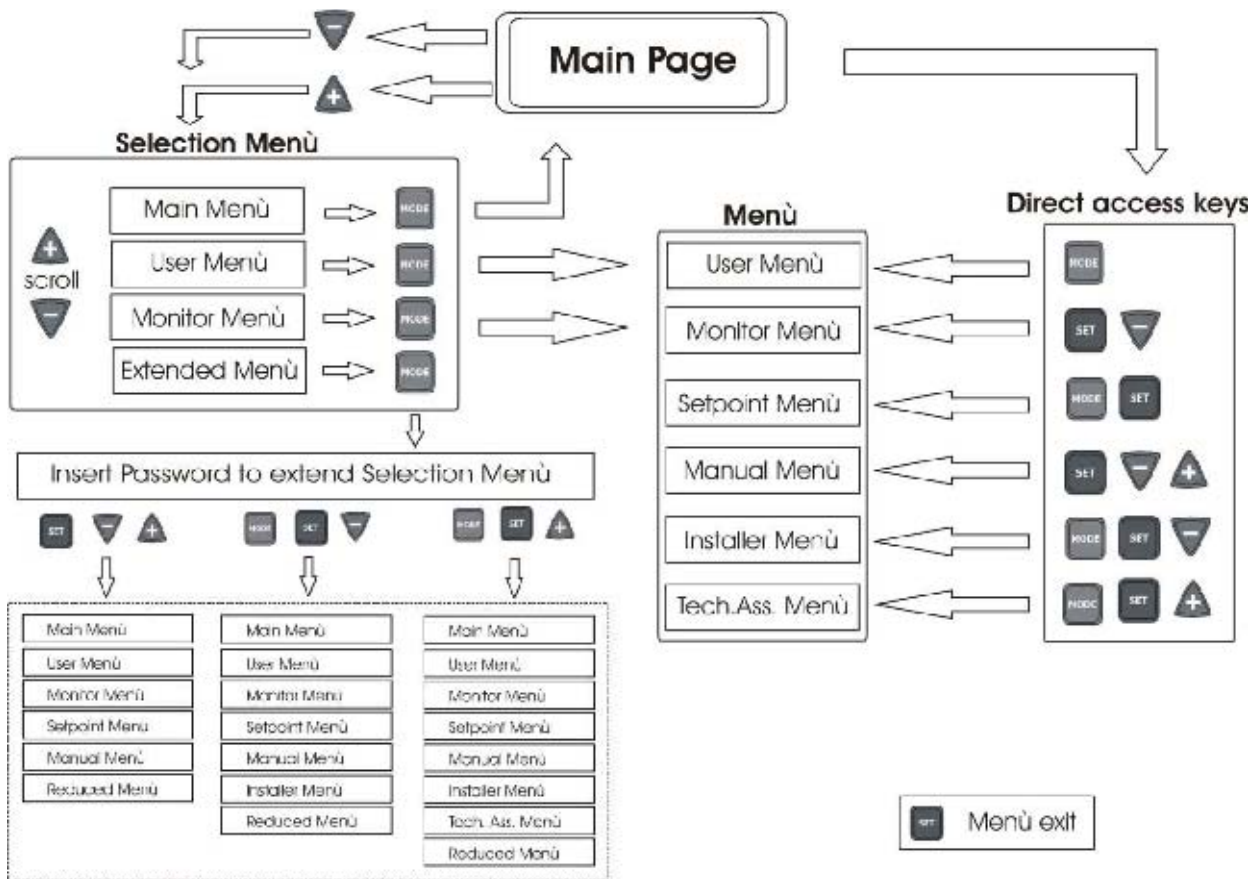
Фигура 14: Схема за достъп
