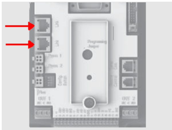
Σχήμα 16: Σύνδεση Link
