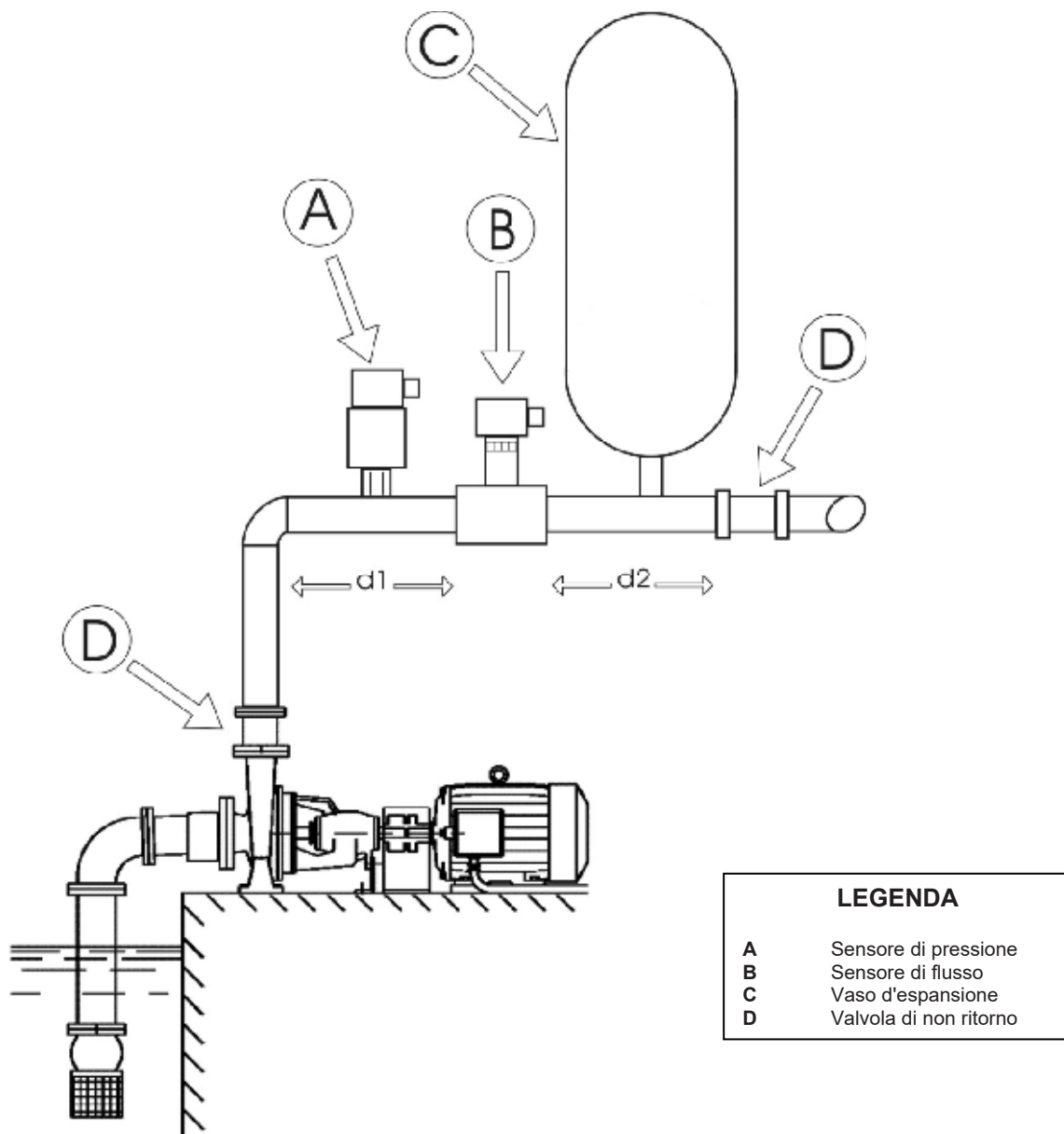
Figura 6: Installazione Idraulica
