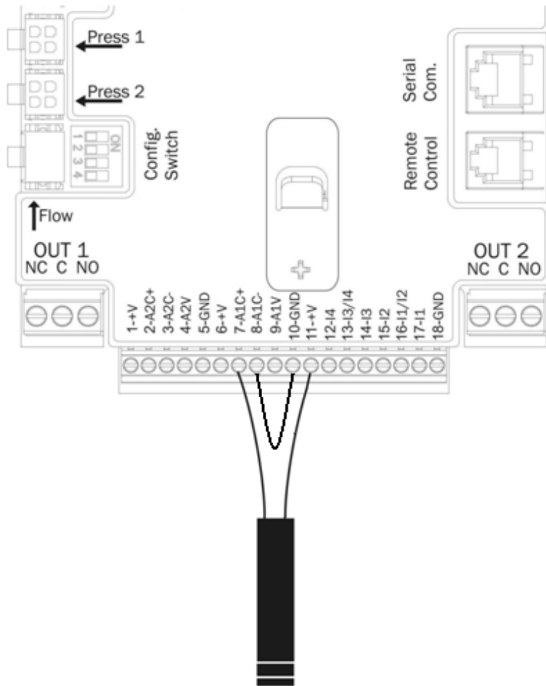
Фигура 8: Свързване на датчик за налягане по ток 4 - 20 мА
