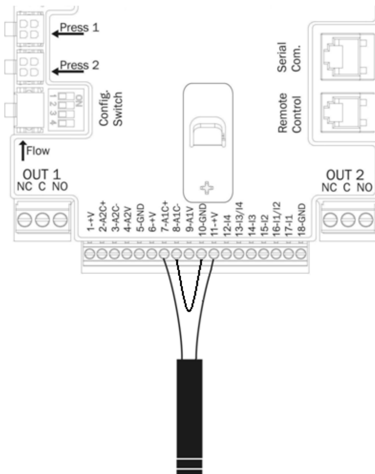
Fig. 8: Anslutning av trycksensor 4 - 20 mA
