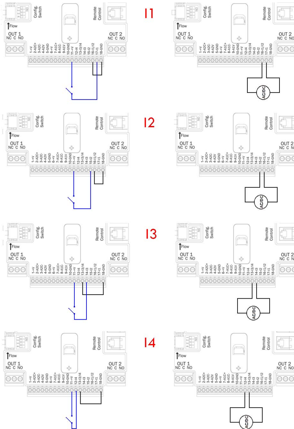
Figura 11: Exemplu de conectare a intrărilor
