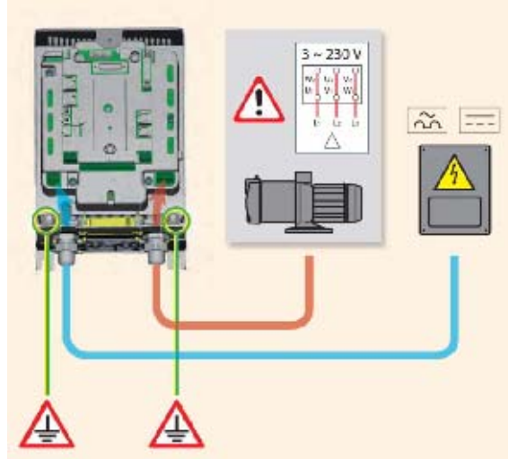
Figura 5: Conexión de la bomba AD 2.2 AC - 1.5 AC - 1.0 AC
