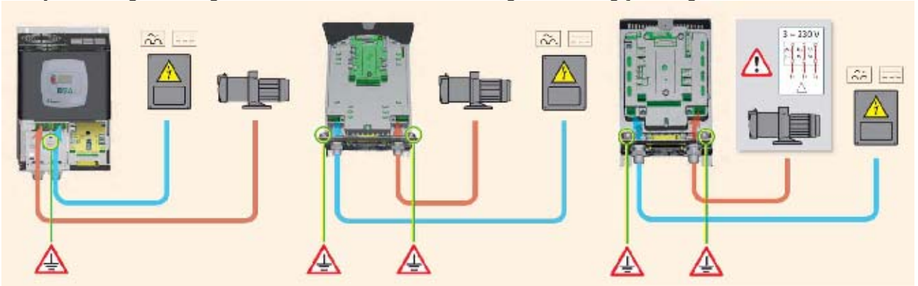
Şekil 4: Elektrik bağlantıları
