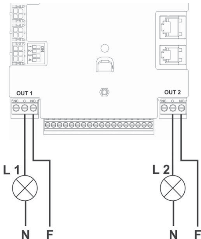
Fig. 10: Exempel på anslutning av utgångar
