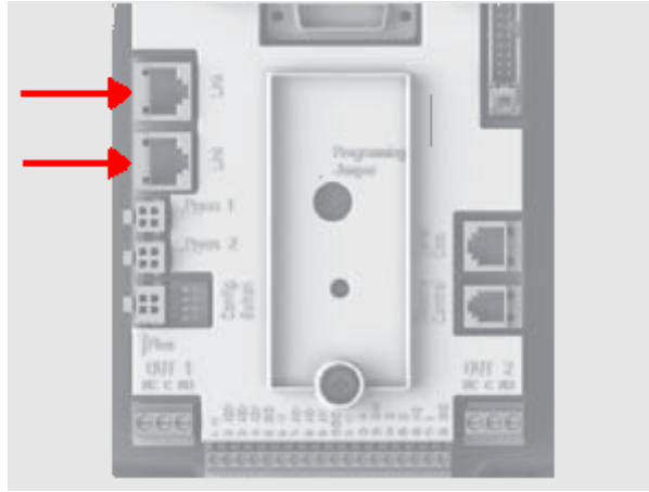
Фигура 16: Линк свързване
