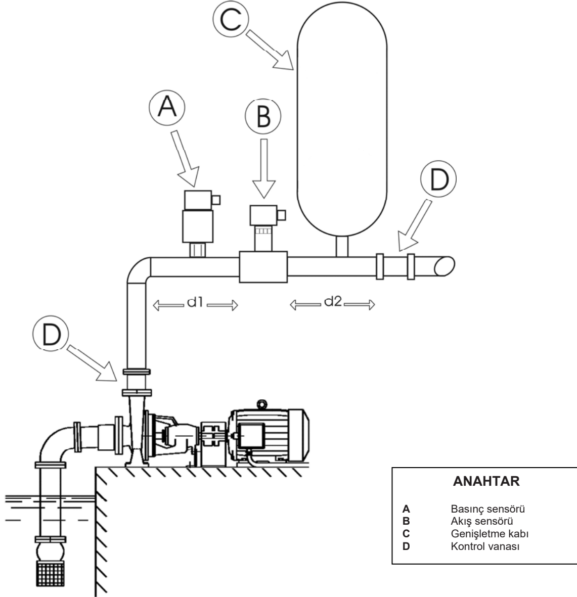
Şekil 6: Hidrolik kurulum
