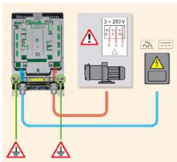
Рисунок 5: Соединение насоса AD 2.2 AC - 1.5 AC - 1.0 AC
