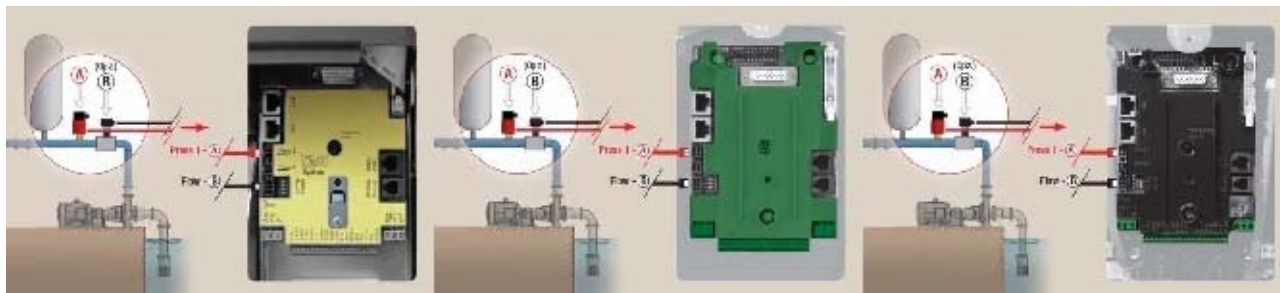
7.ábra: A szenzorok bekötése
