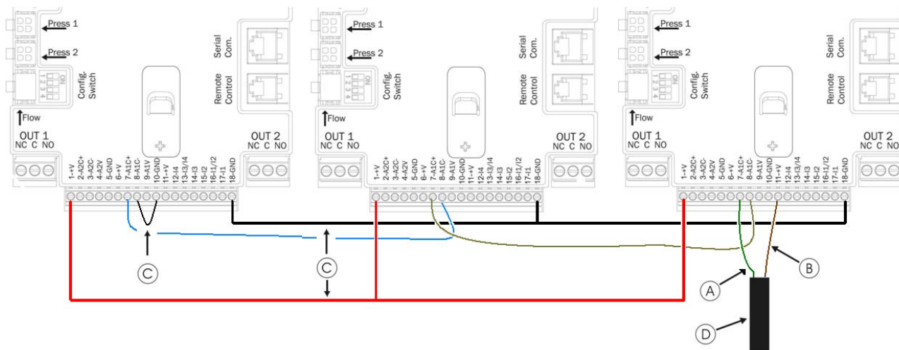
9. ábra: A 4-20mA-es nyomás szenzor bekötése egy multi inverteres rendszerbe
