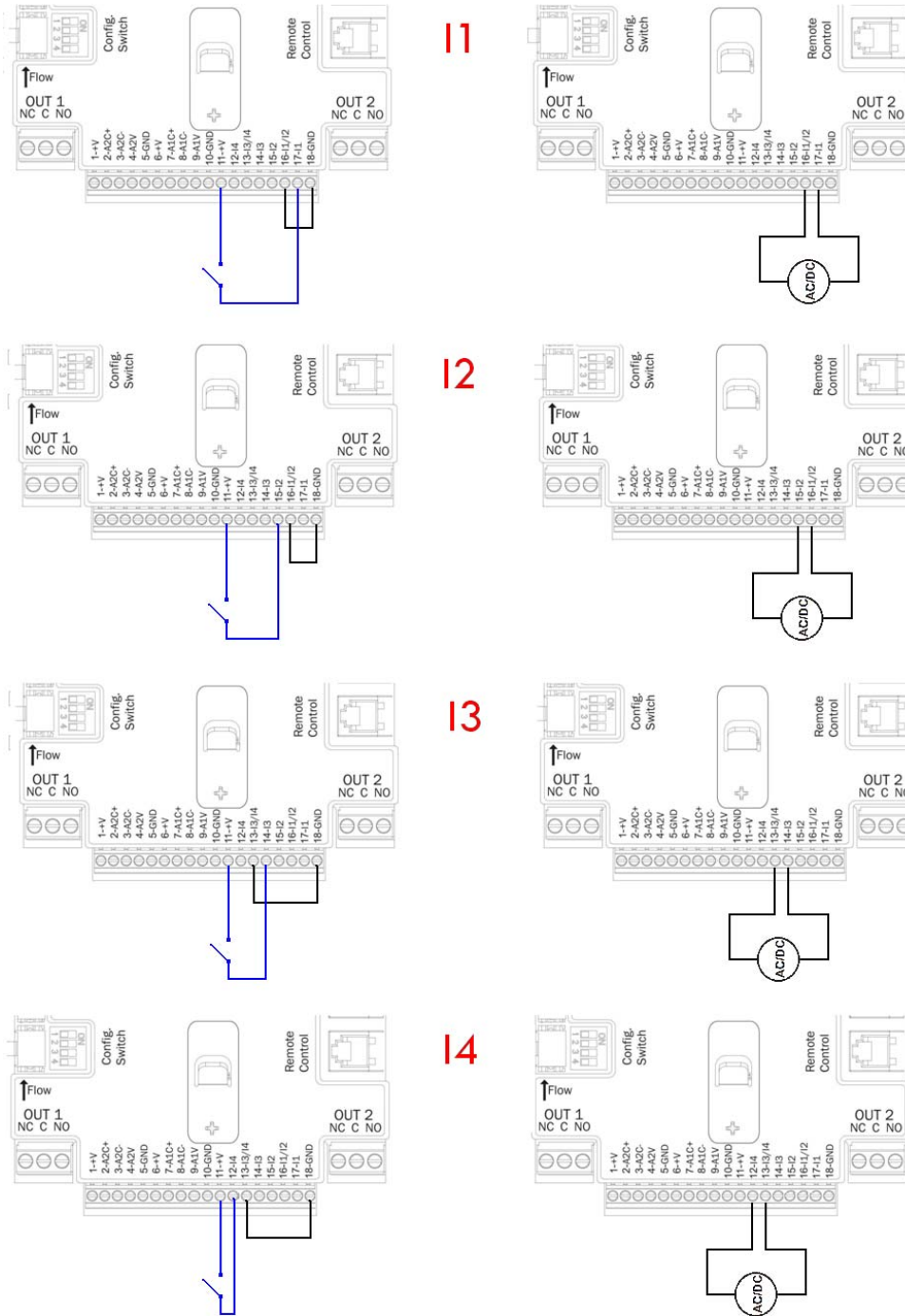
11.ábra: Példa a bemenetek bekötésére
