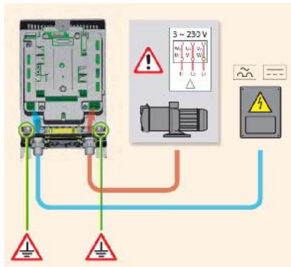
Abbildung 5: Anschluss Pumpe AD 2.2 AC - 1.5 AC - 1.0 AC
