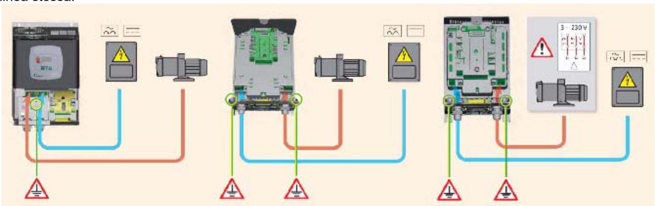
Figura 4: Connessioni elettriche
