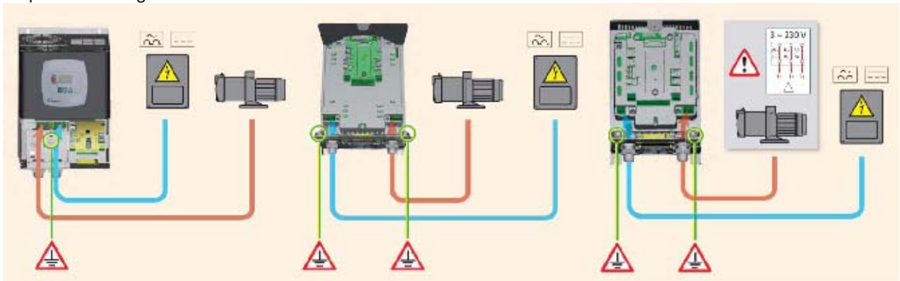
Figure 4: Connexions électriques
