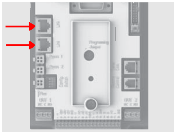
Figura 16: Conectarea Link
