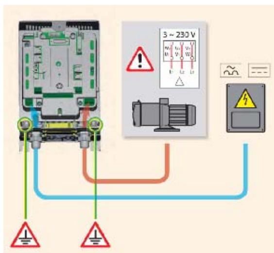
Σχήμα 5: Σύνδεση αντλίας AD 2.2 AC - 1.5 AC - 1.0 AC
