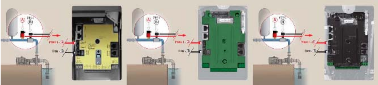
Afbeelding 7: Aansluitingen sensoren
