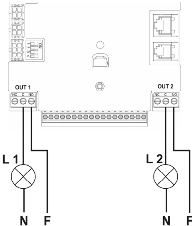
Фигура 10: Пример на свързване на изхода
