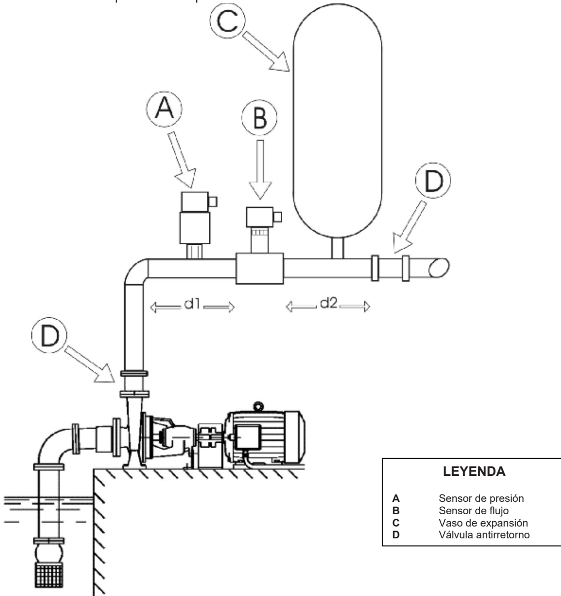
Figura 6: Instalación hidráulica
