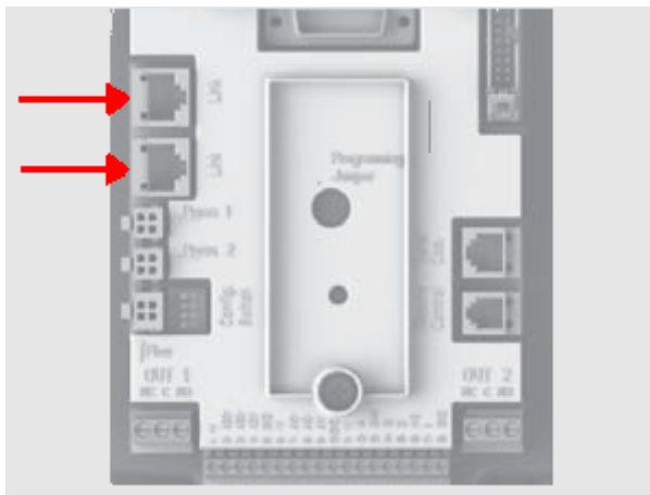
Figura 16: Connessione Link
