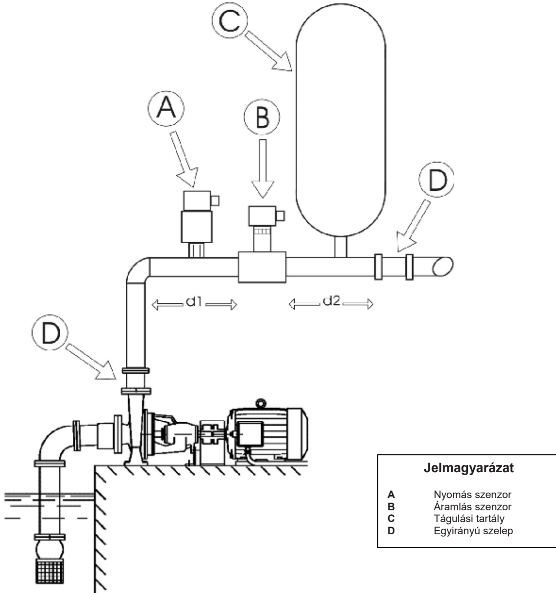
6.ábra: Hidraulikus installáció
