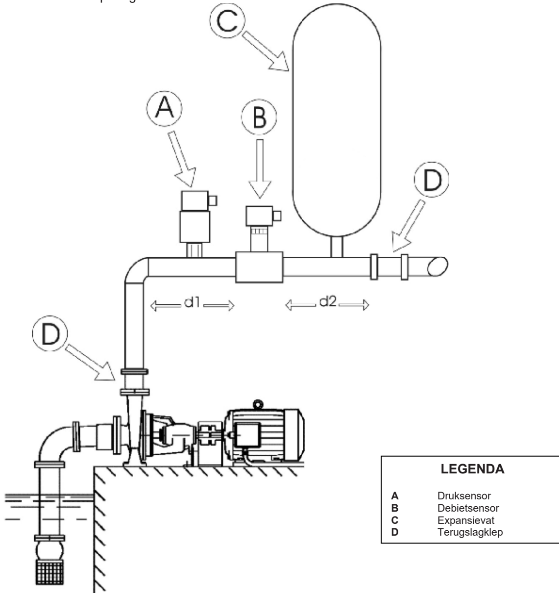
Afbeelding 6: Hydraulische installatie
