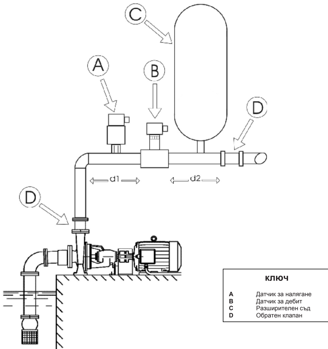
Фигура 6: Хидравлична схема
