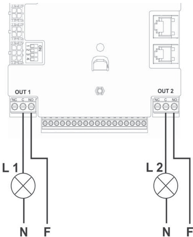
Figura 10: Ejemplo de conexión de las salidas
