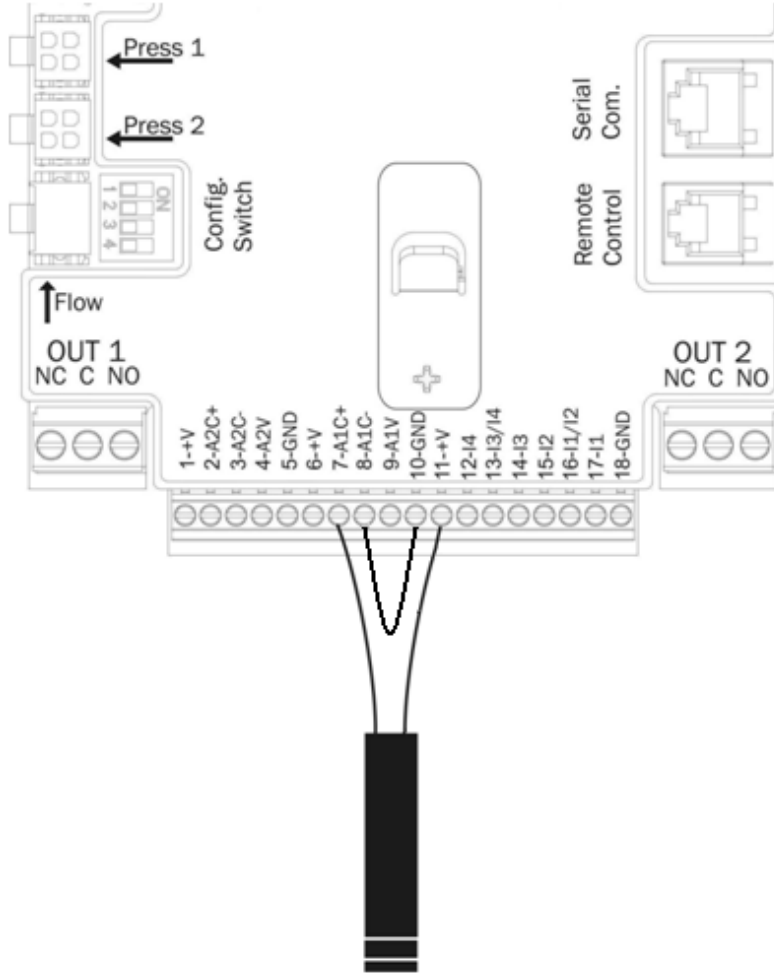
Şekil 8: 4 - 20 mA basınç sensörünü bağlama
