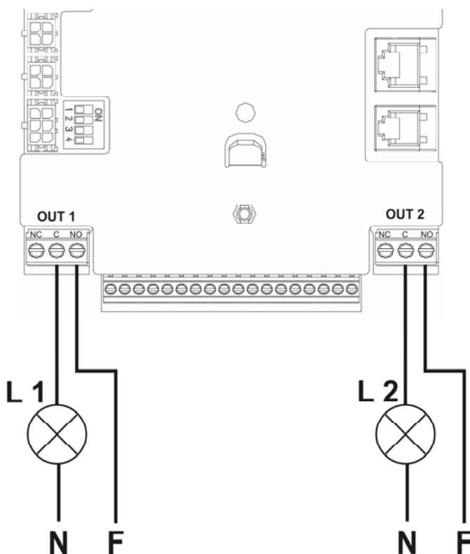
10.ábra: Példa kimenetek bekötésére
