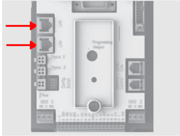
Fig. 16: Kommunikationskabel
