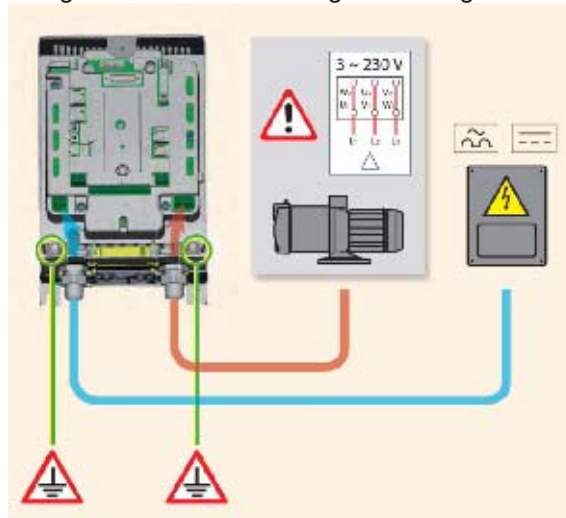
Figura 5: Conectarea pompei AD 2.2 AC - 1.5 AC - 1.0 AC
