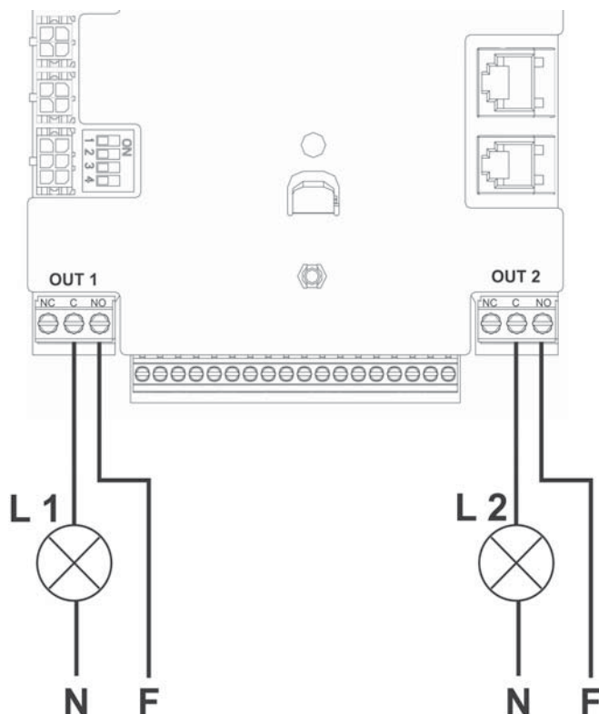
Figura 10: Exemplu de conectare a ieșirilor
