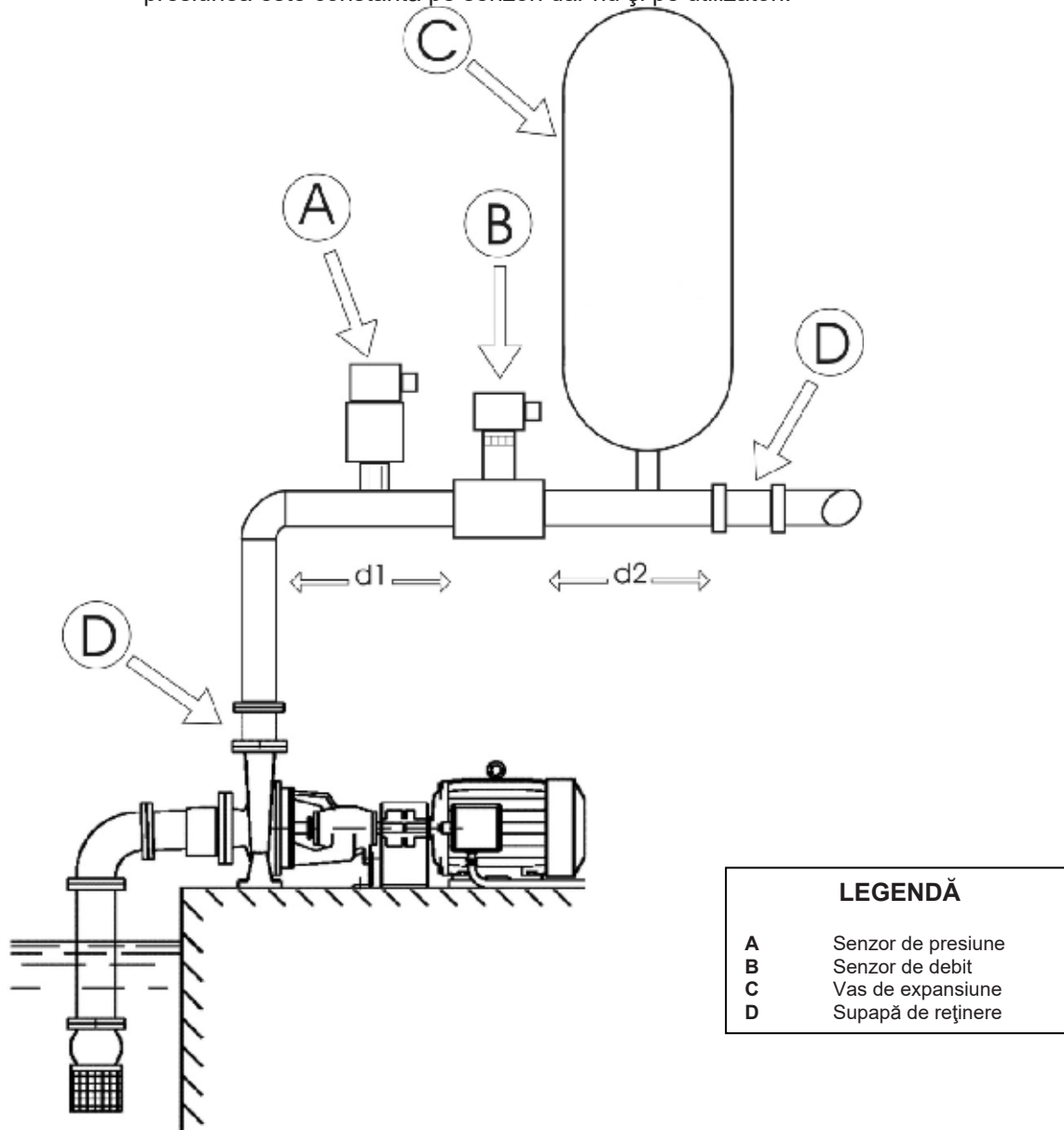
Figura 6: Instalația hidraulică
