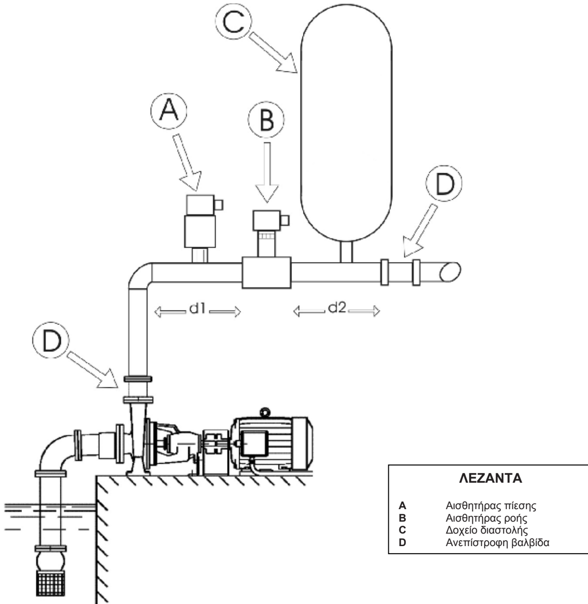
Σχήμα 6: Υδραυλική εγκατάσταση
