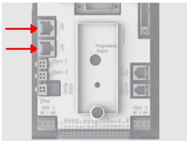
Рисунок 16: Соединение Link
