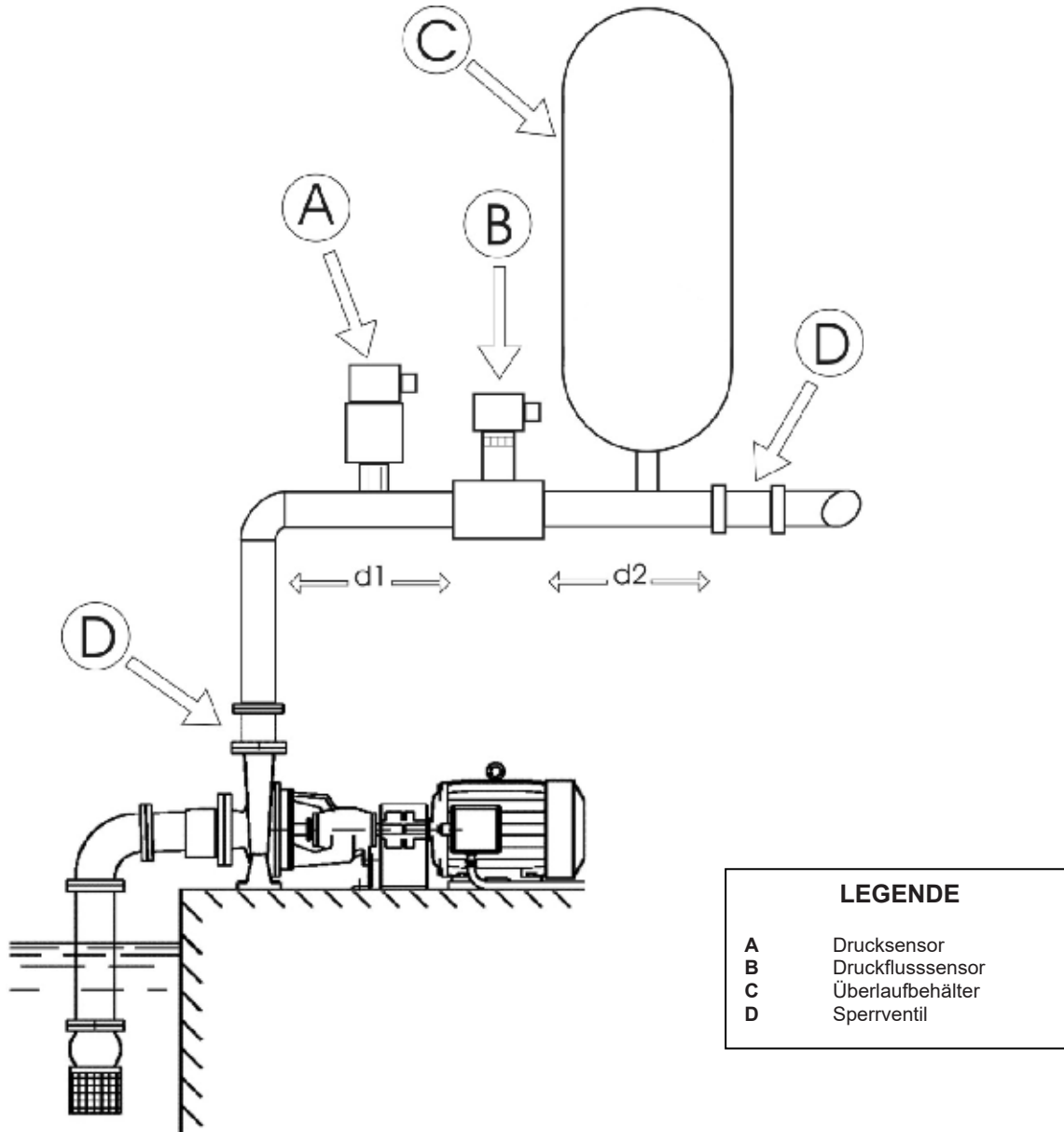
Abbildung 6: Hydraulik-Installation
