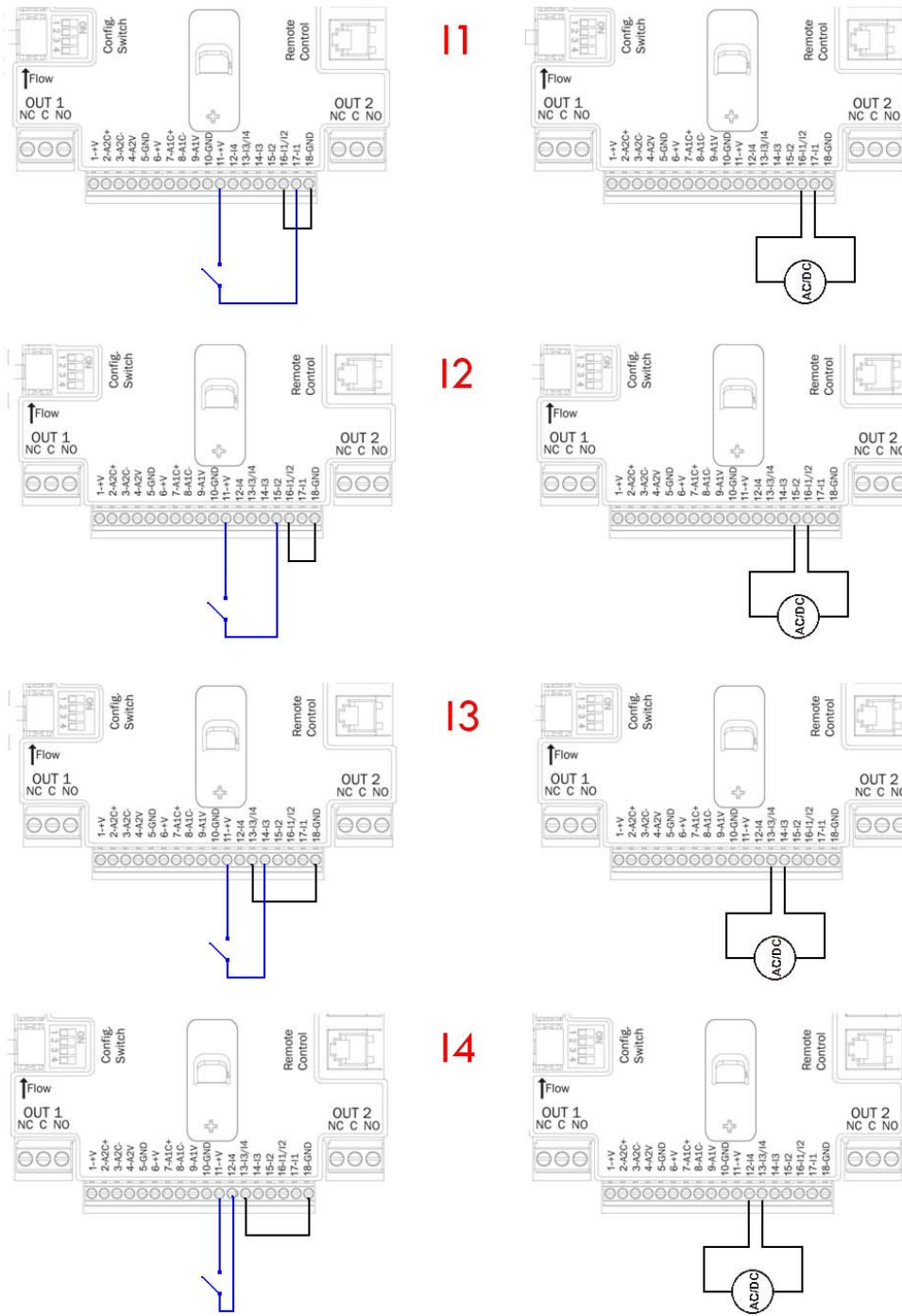
Figure 11: Exemple de connexion des entrées
