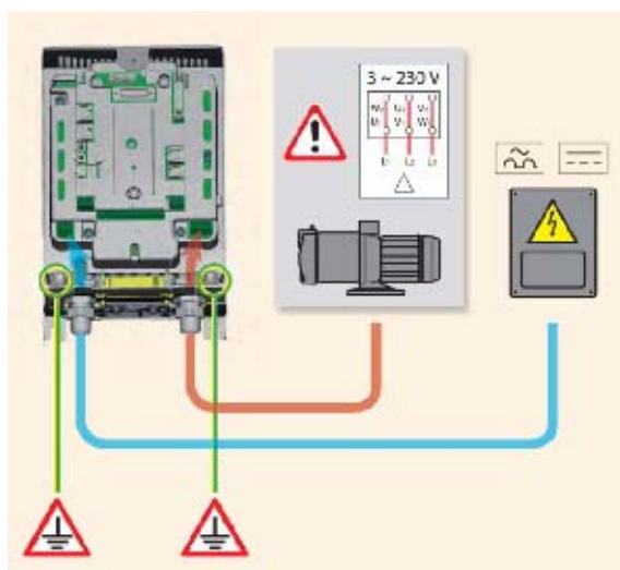
Figura 5: Collegamento pompa AD 2.2 AC - 1.5 AC - 1.0 AC
