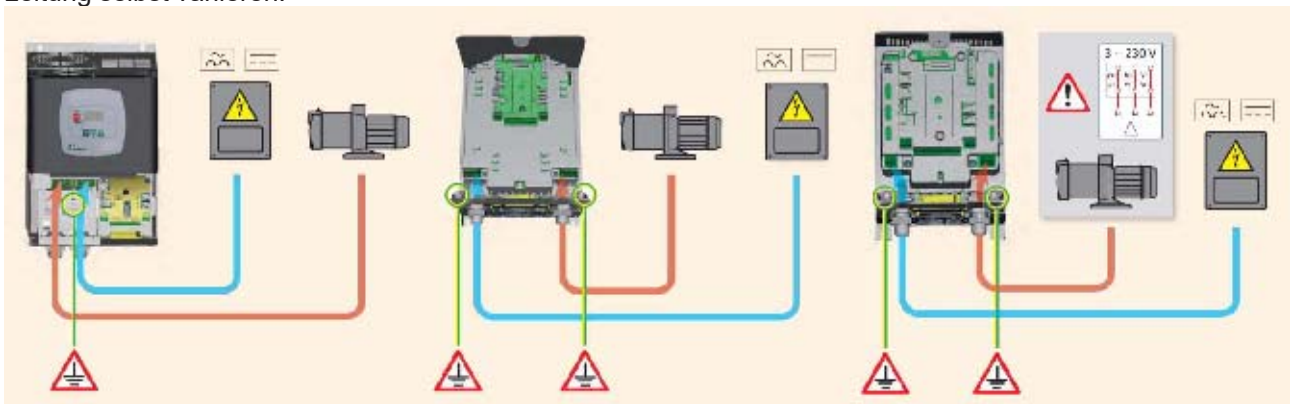
Abbildung 4: Elektrische Anschlüsse
