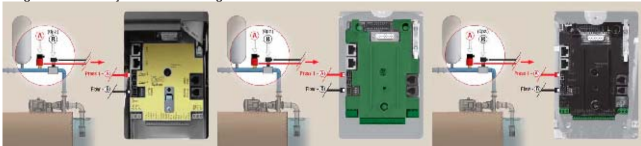
Figura 7: Conexiuni senzori
