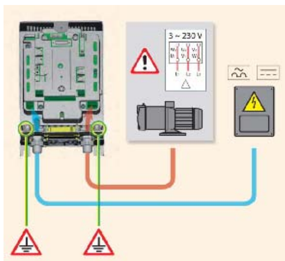
Фигура 5: Свързване на помпа AD 2.2 AC - 1.5 AC - 1.0 AC
