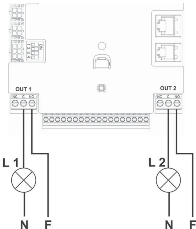
Рисунок 10: Пример соединений выходов
