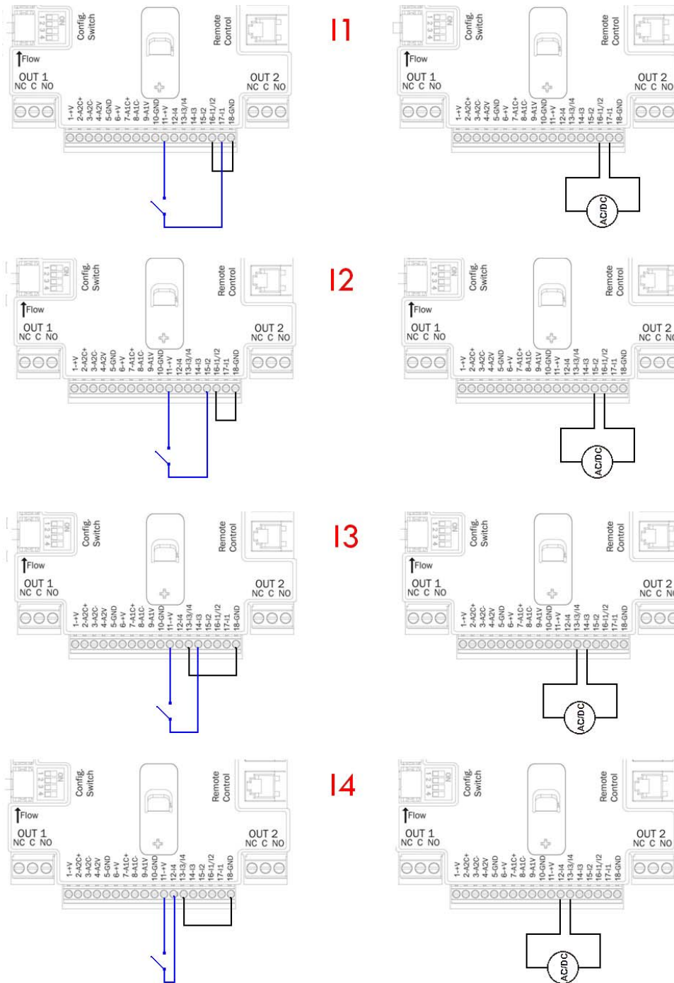
Фигура 11: Пример на свързване на входа
