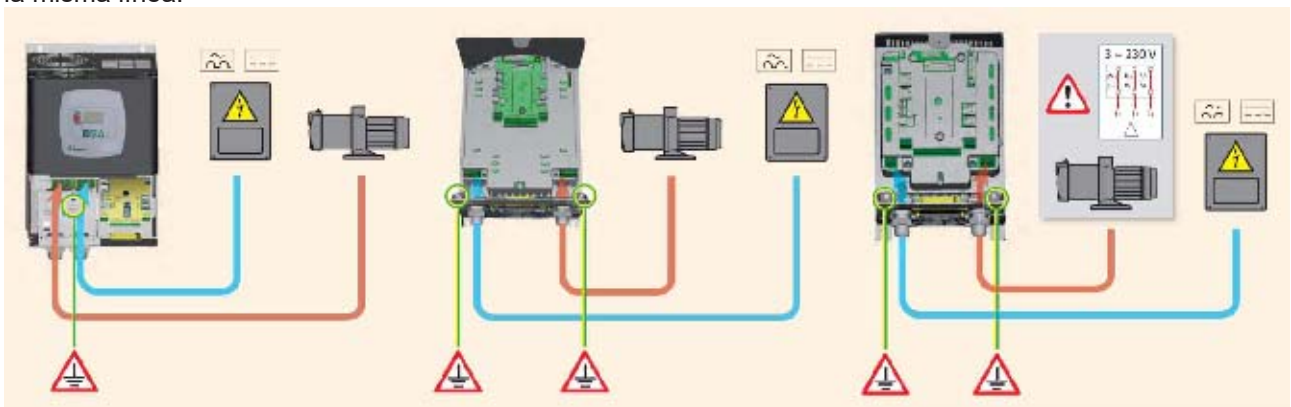
Figura 4: Conexiones eléctricas
