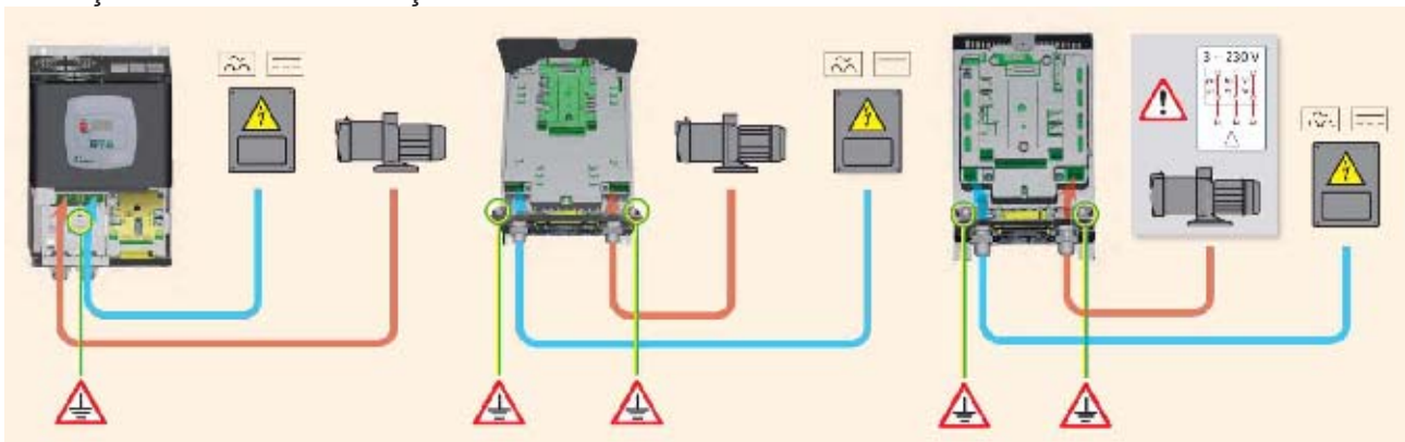
Figura 4: Conectări electrice
