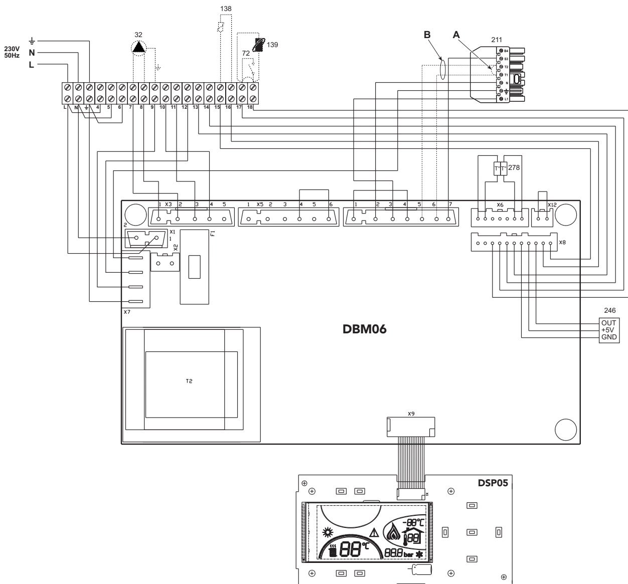
рис. 18 - Электрическая схема
