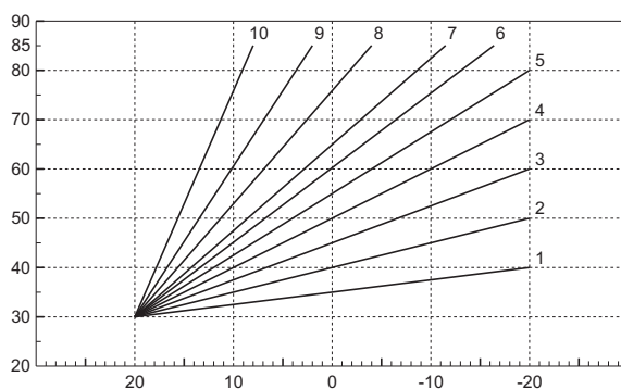
рис. 11 - Компенсационные характеристики
