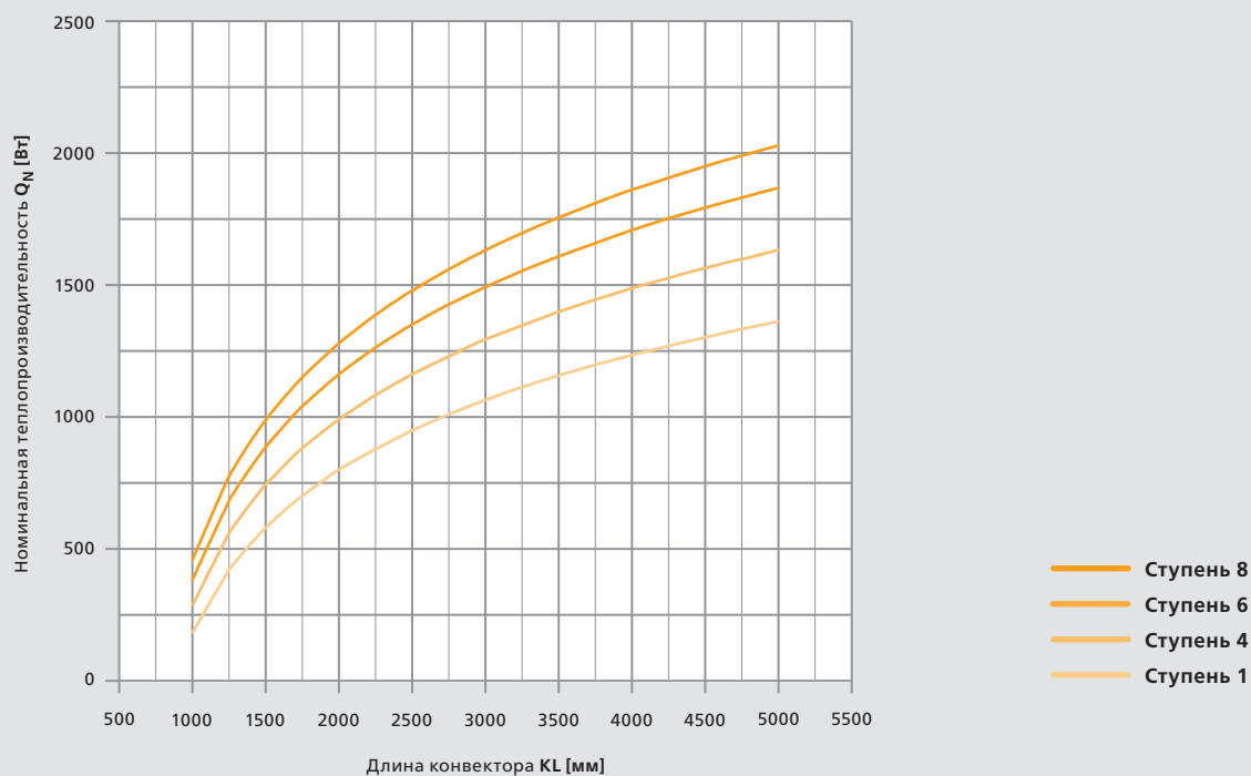
Номин.теплопроизвод. Q_N [Вт] при различных ступенях вентилятора и \Delta T = 50K
