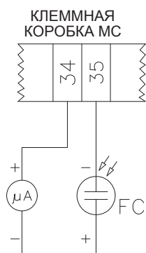
Рис. 21 - Контроль пламени с помощью фотоэлемента QRA.
