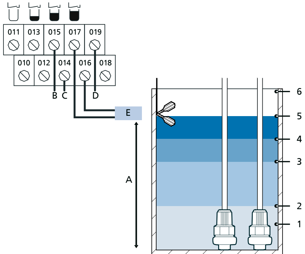
Рисунок 24: Двойная насосная станция: Опорожнение при аналоговом измерении 4 .. 20 мА
