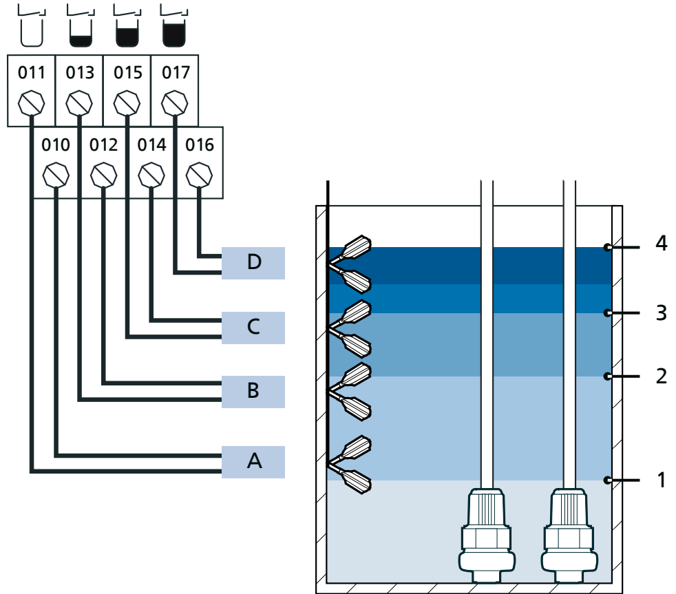
Рисунок 18: Двойная насосная станция: Опорожнение посредством трех поплавковых выключателей (без гистерезиса)
