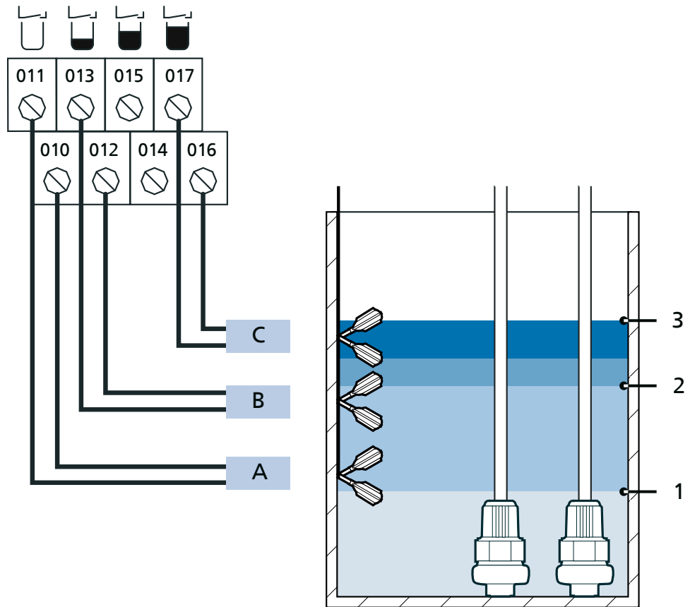
Рисунок 19: Двойная насосная станция в качестве резервного насоса: Опорожнение посредством двух поплавковых выключателей (без гистерезиса)
