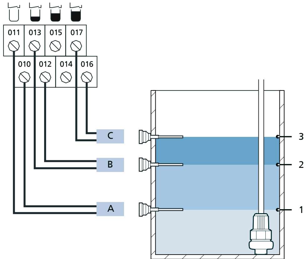
Рисунок 14: Одиночная насосная станция: Опорожнение посредством 2 цифр. реле уровня
