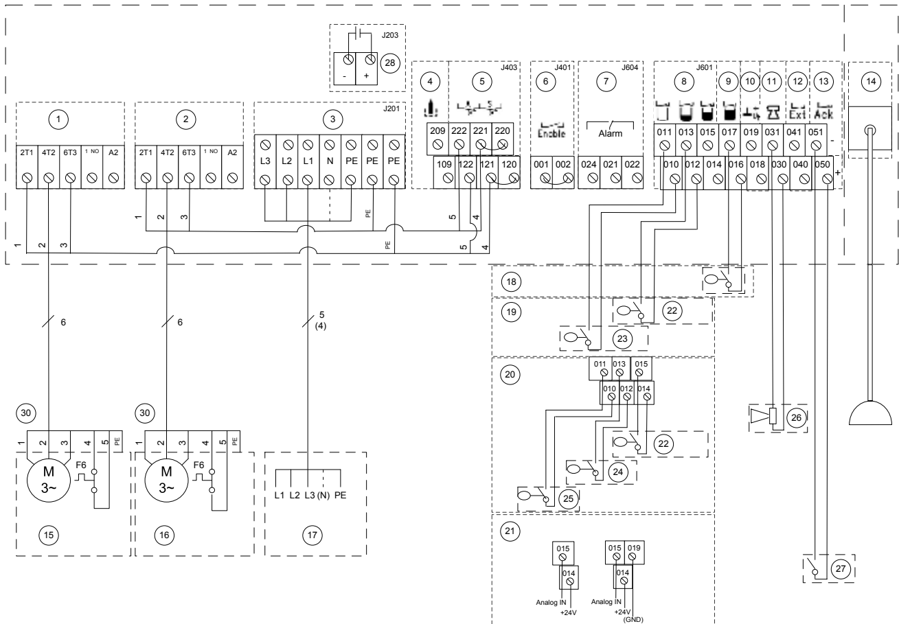
Рисунок 33: Схема электрических соединений Ama-Drainer V(80)
