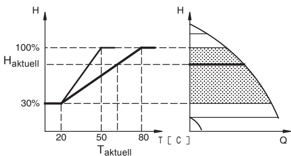
Рис. 13 Регулирование по температуре
