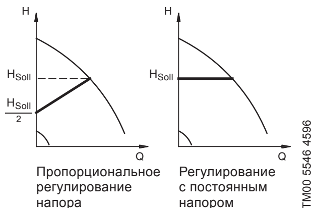
Рис. 10 Регулирование напора
