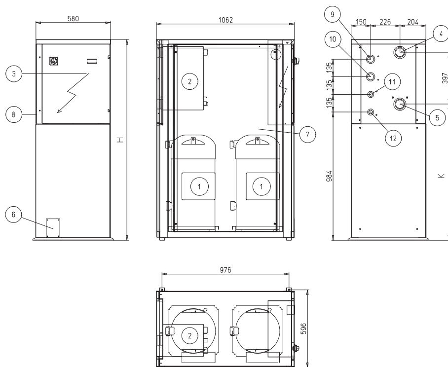
Чертеж №2 (ME 292÷422)
