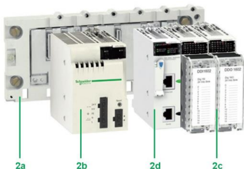
Платформа ввода/вывода Modicon X80
