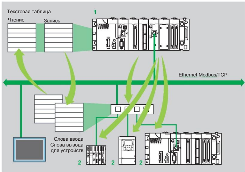
2 Устройство с обменом сообщениями Modbus TCP в режиме сервера
