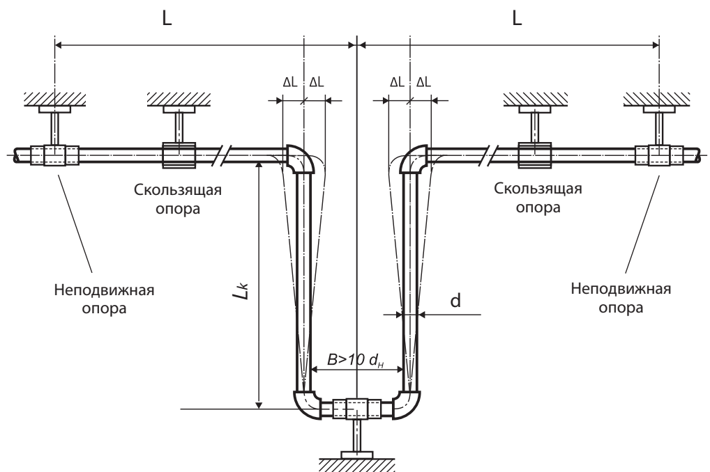
Рис. 10. П-образный компенсатор
