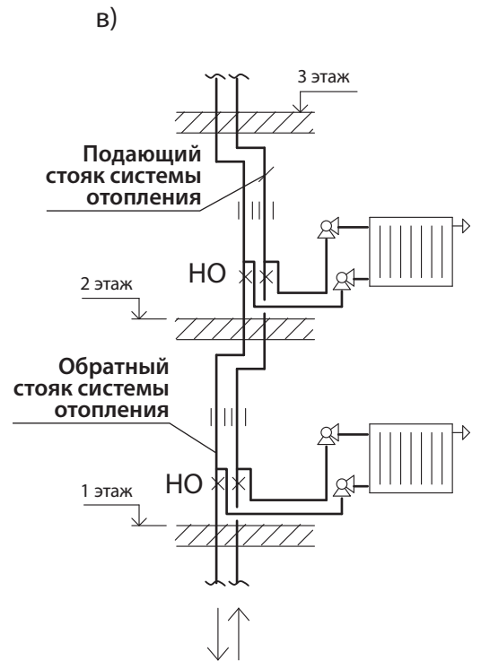
Рис. 14. Примеры расстановки неподвижных опор и компенсаторов на стояках систем отопления из многослойных напорных полипропиленовых труб, армированных стекловолокном или алюминиевой фольгой
