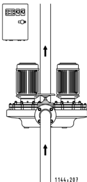
Крепление Trialine Z типоразмеров ...-160/... и ...-250/... с 3 опорными лапами (см. Принадлежности)
