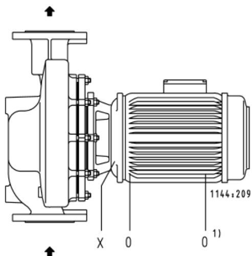
Горизонтальный монтаж, направление потока снизу вверх.
