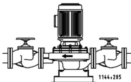
Крепление Trialine Z типоразмеров ...-160/... и ...-250/... с 3 опорными лапами (см. Принадлежности)
