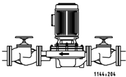
Крепление Trialine Z без опорных лап
