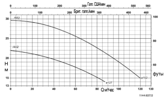
Trialine Z 65-160
