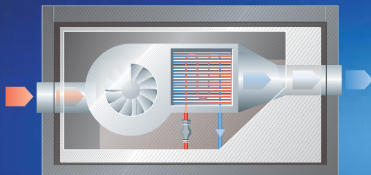
Modul Abluft
