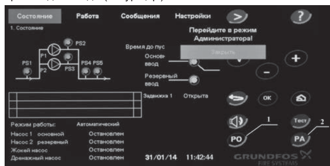
10-сур. «РА» түймесін басудан кейін оператор панелінің экраны
