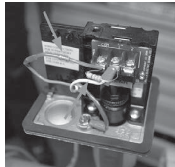
Նկար 3 Ճնշման ռելեի հենամարմնում դիմադրությունների (ռեզիստորների) տեղադրման օրինակ
