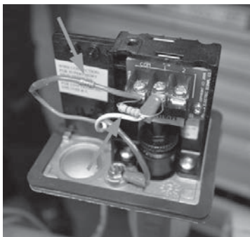
3-сүр. Басым релесинин корпусунда каршылыктарды (резисторлорду) орнотуу мисалы
