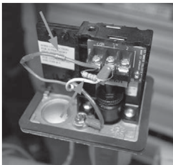
3-сур. Қысым релесі корпусына кедергілерді (резисторлар) орнату мысалы
