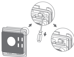
Рисунок 16. Демонтаж опорной пластины терморегулятора
