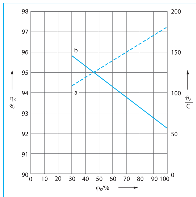
14/3 Температура дымовых газов и коэффициент полезного действия чугунного отопительного Ecostream-котла Logano GE615 при средней температуре котловой воды 70 °С
