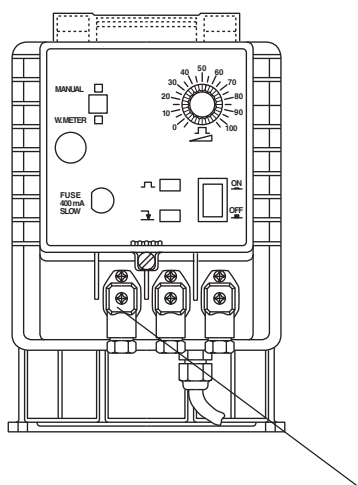
Подключение контактного водосчетчика
