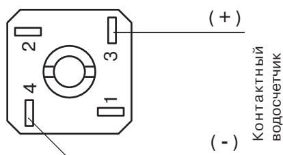
Подключение контактного водосчетчика
