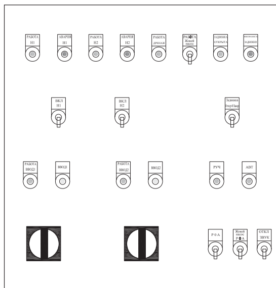
Рис. 1 Шкаф управления пожарными насосами. Внешний вид.
