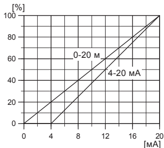
Рис. 11. Масштабирование аналогового сигнала с положительным углом наклона
