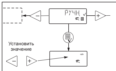
Рис. 9. Алгоритм установки производительности насоса
