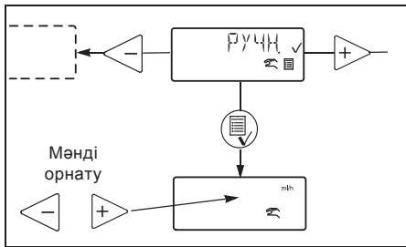
9-сур. Сорғы өндірімділігін орнату алгоритмі
