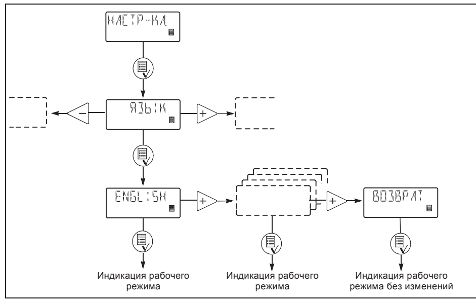
Рис. 23. Алгоритм выбора языка
