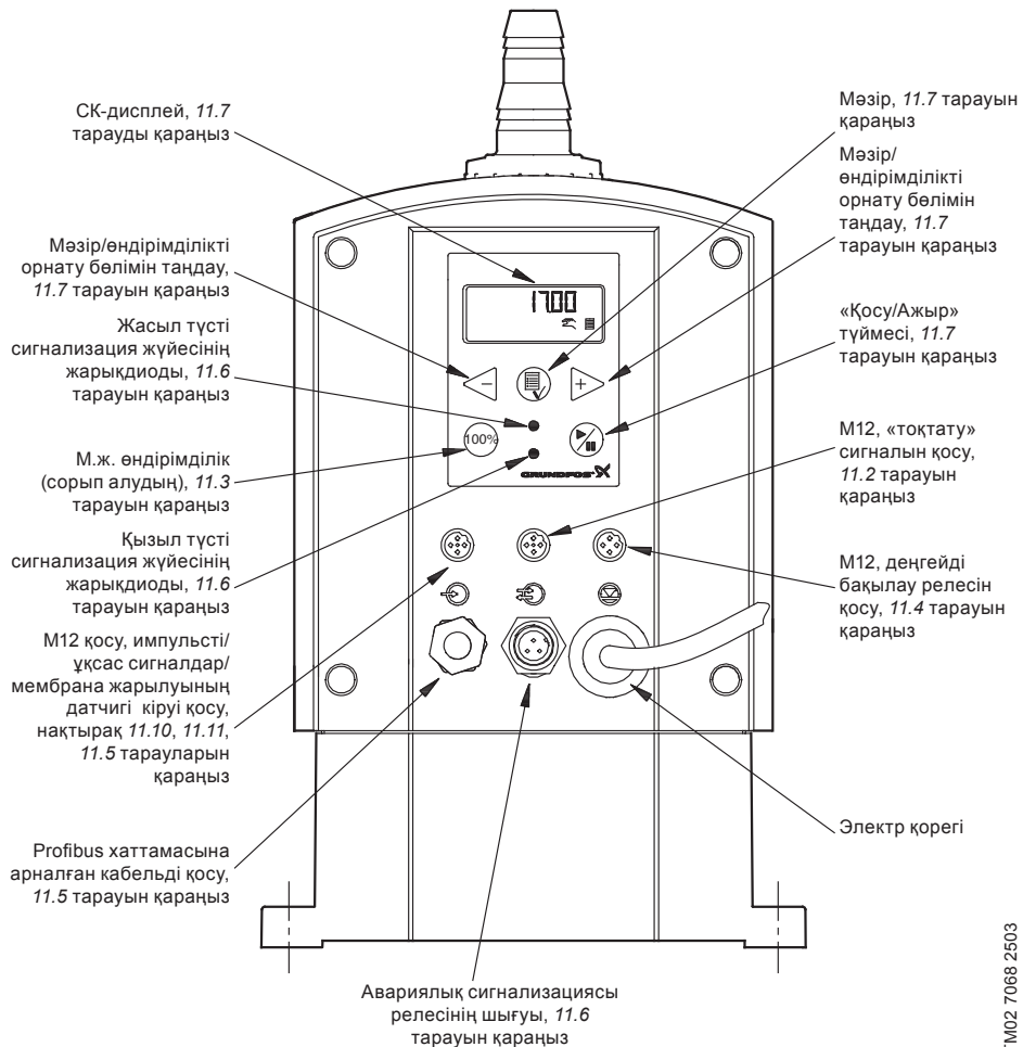
7-сур. DME сорғысы, алдығы жағындағы кескіні
