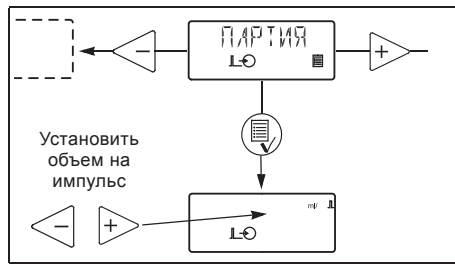
Рис. 17. Алгоритм установки режима работы - «Партия»
