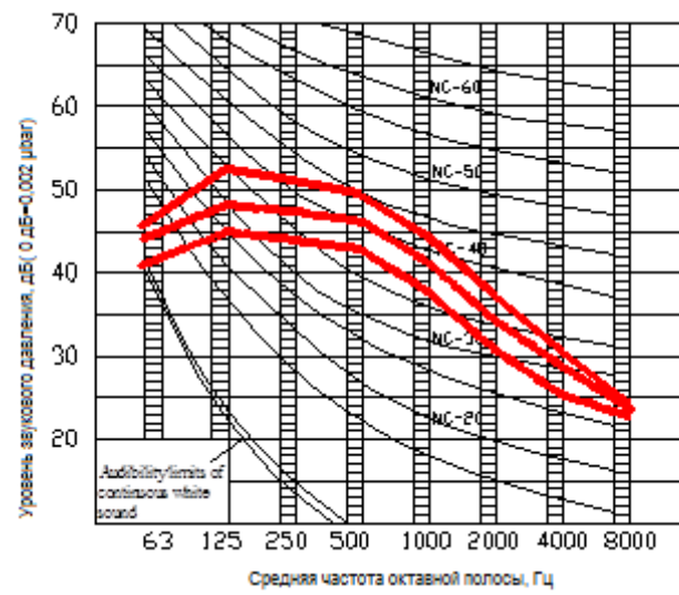
MVC140A-VA1
