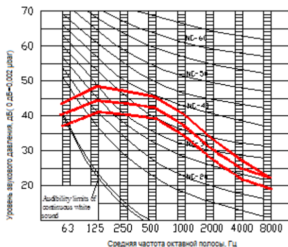
MVC71(80)A-VA1
