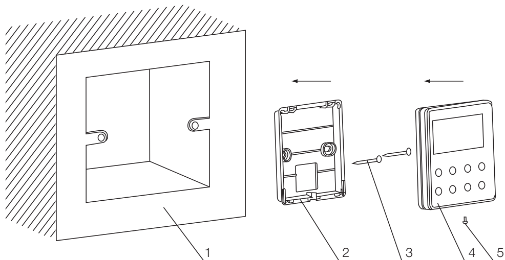
Схема установки проводного пульта
