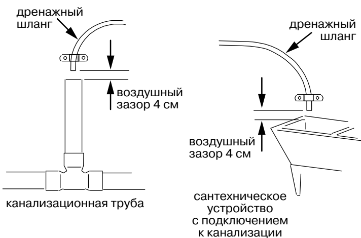
Рис. 3. Подключение дренажа
