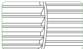
Смещенное расположение лопаток рабочего колеса для снижения шума.
