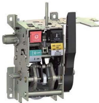
Рабочий механизм
