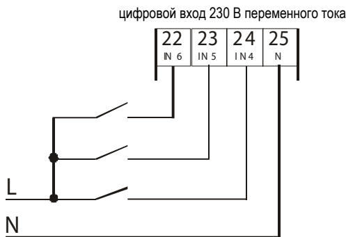
Схема подключения цифровых входов 230 В переменного тока
