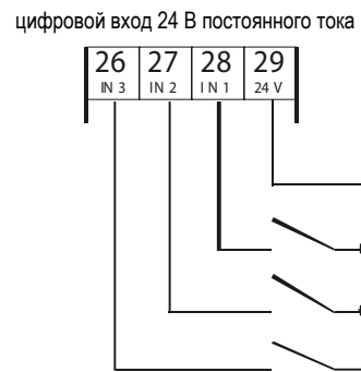
Схема подключения цифровых входов 24 В постоянного тока
